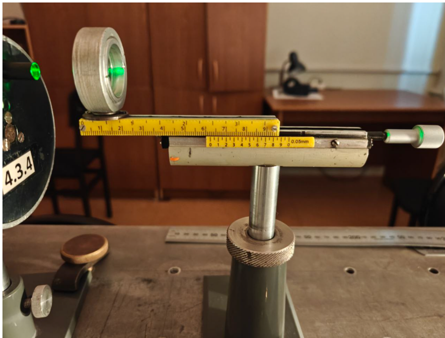
Рис. 1. Отсчёт по шкале микровинта. Значение снималось по вертикальной риске корпуса.
