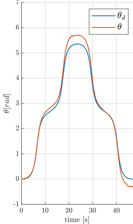
Desired VS Actual orientation
