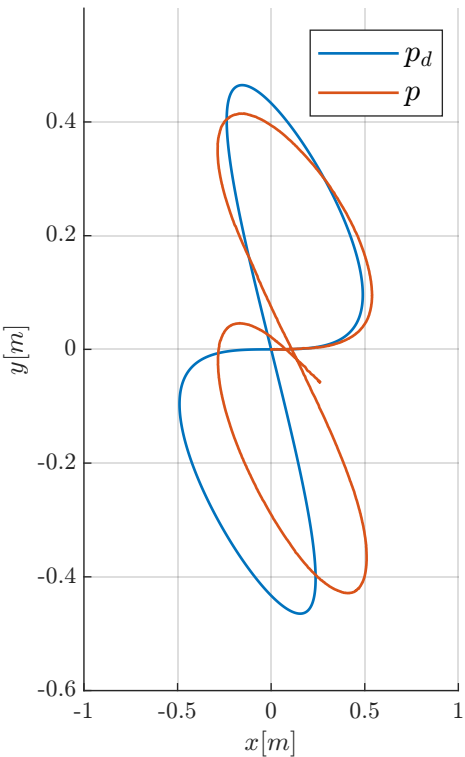
Desired VS Actual position
