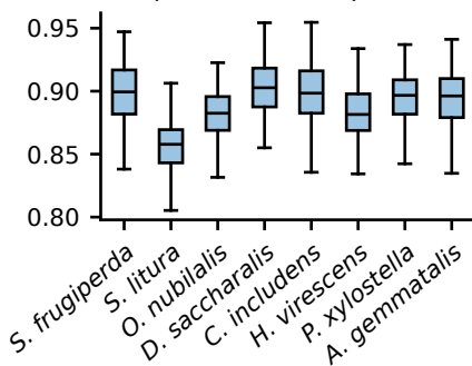
pLDDT do complexo
