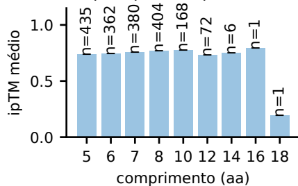
ipTM por comprimento
