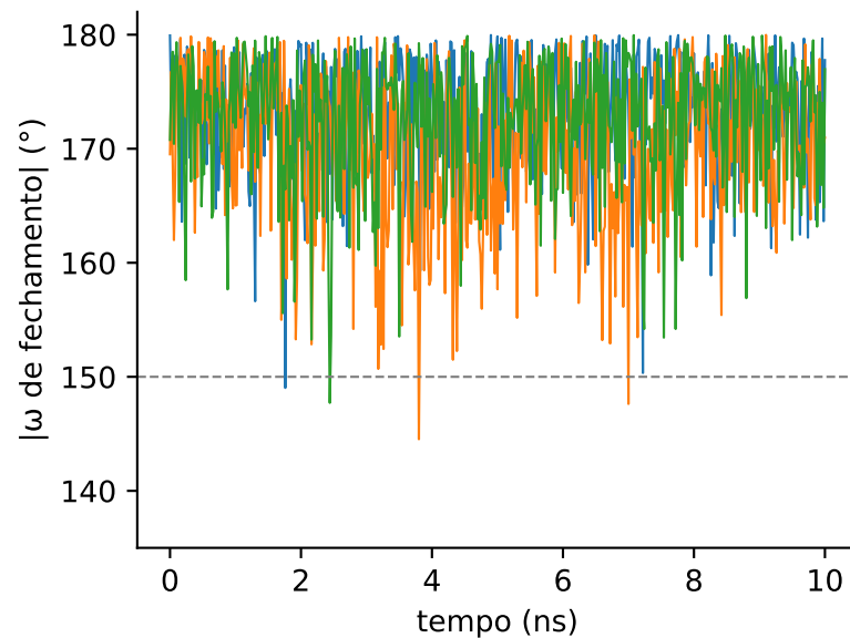
Integridade do anel nas simulações cíclicas com CHARMM36 (tracejado: limites pré-registrados, C-N \leq 1,5 \text{ \AA} e \omega \geq 150^\circ )
