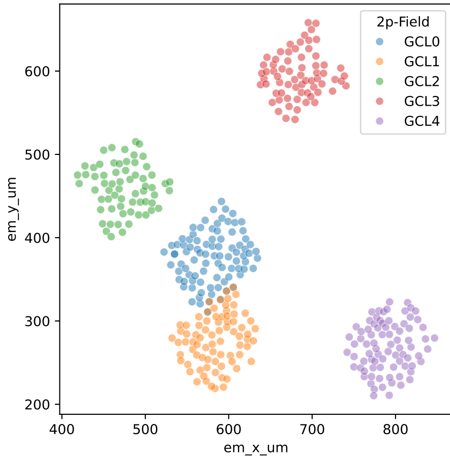
EM coordinates (reference)
