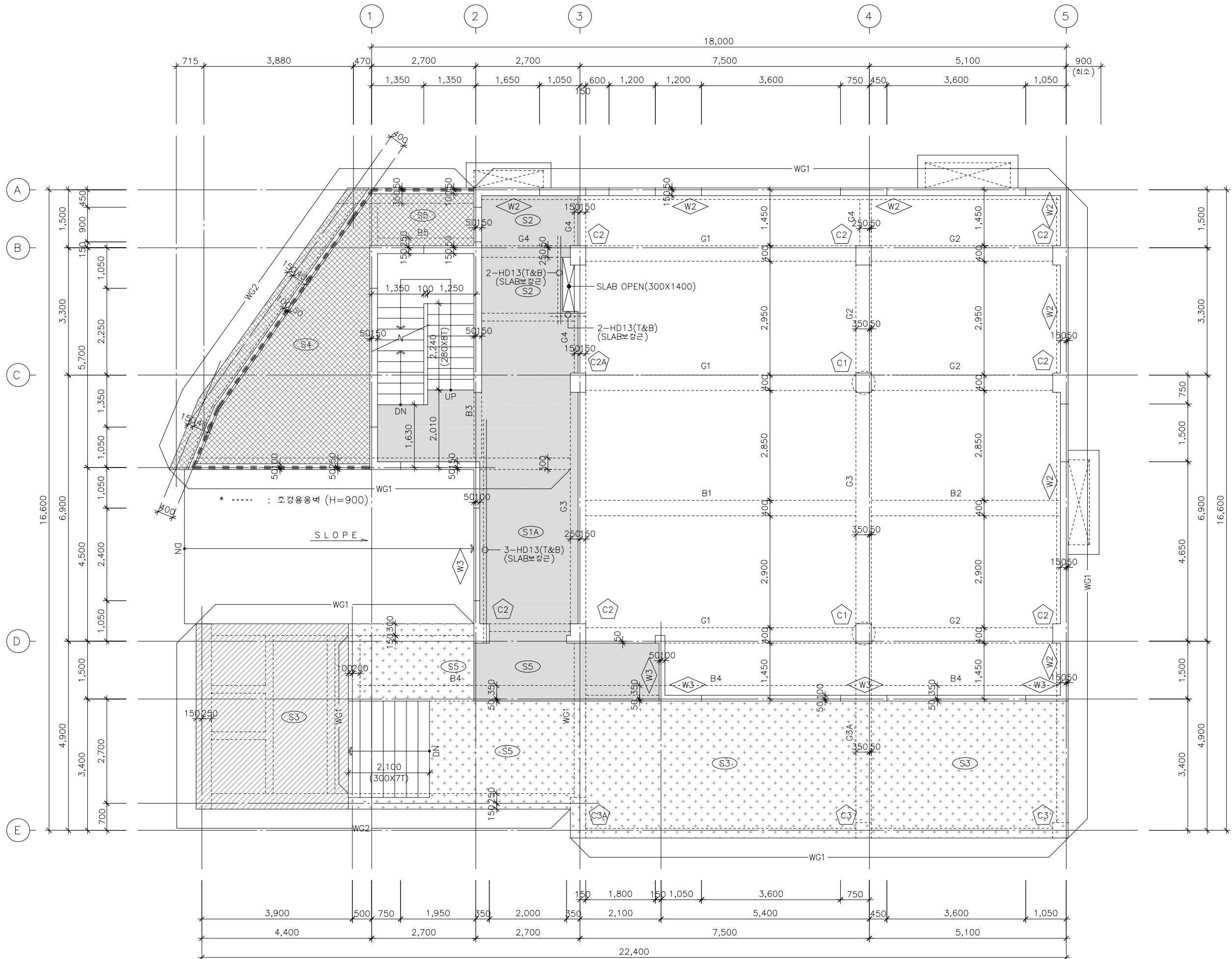
1층 구조 평면도 축척 : 1/100
