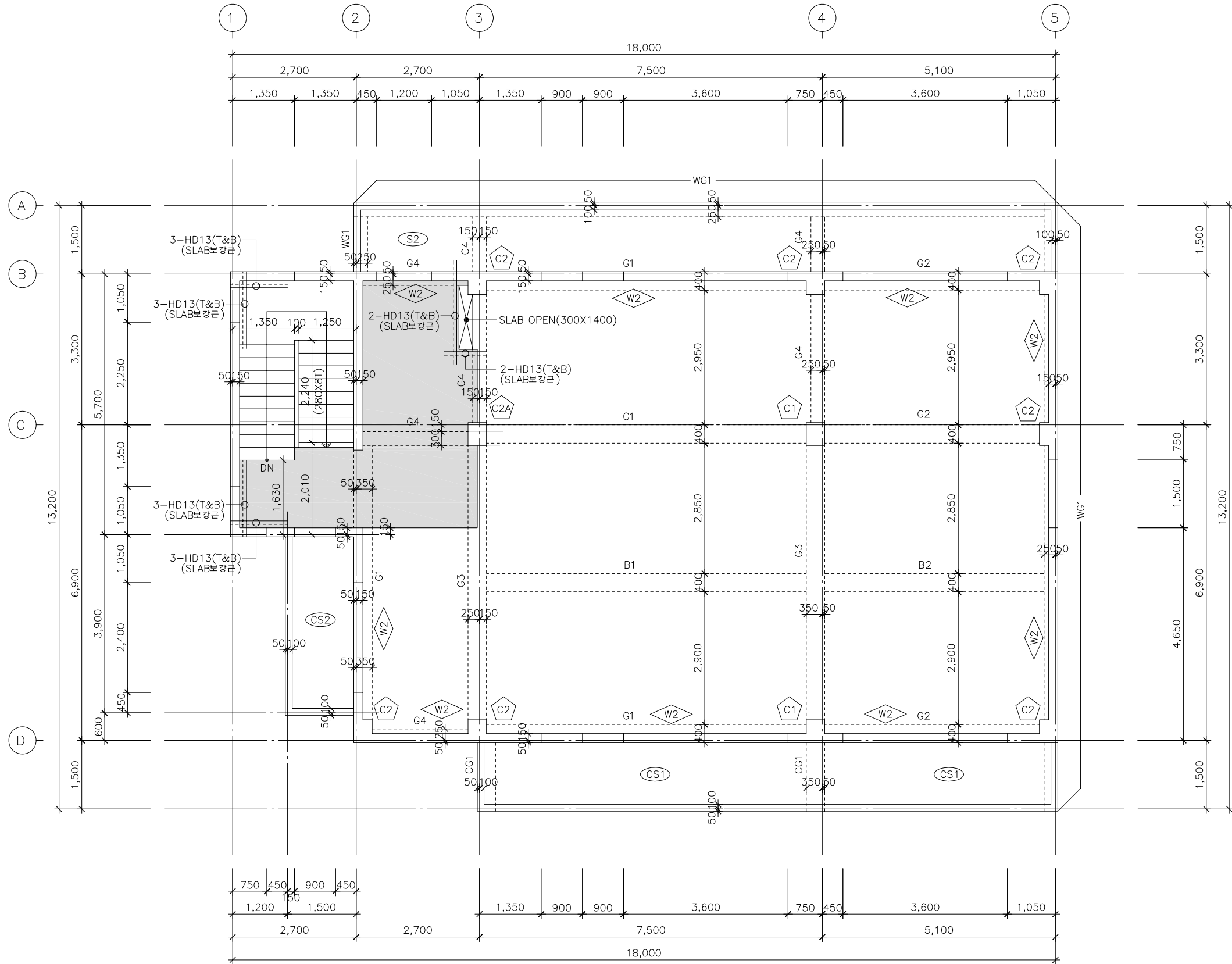
1 3층 구조 평면도 축척 : 1/100
