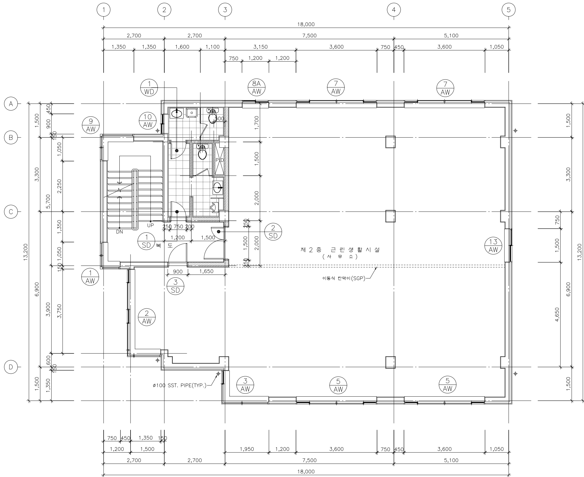
1 2층 평면도 A - 축척 : 1/100
