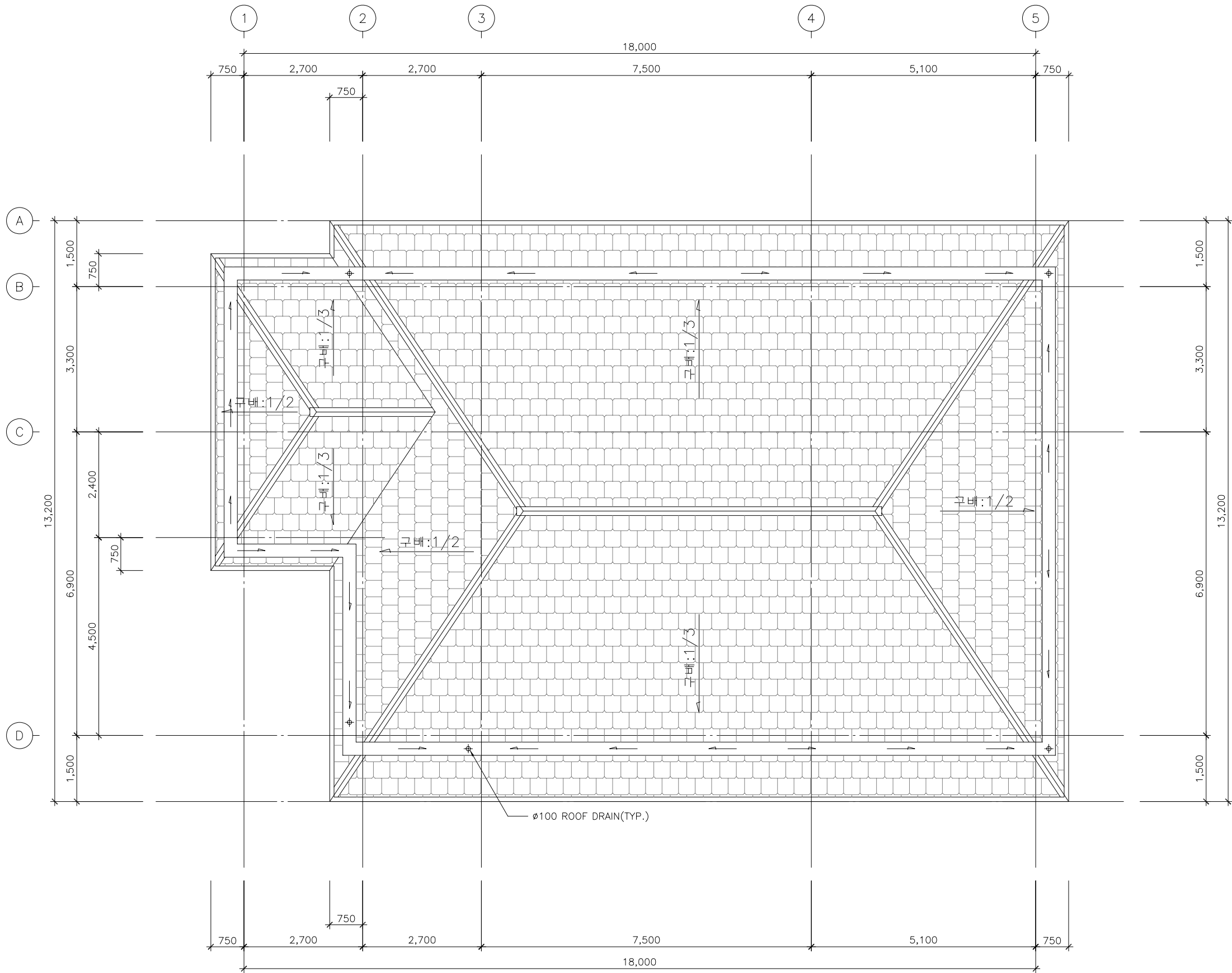
1 지붕 평면도 축척 : 1/100
