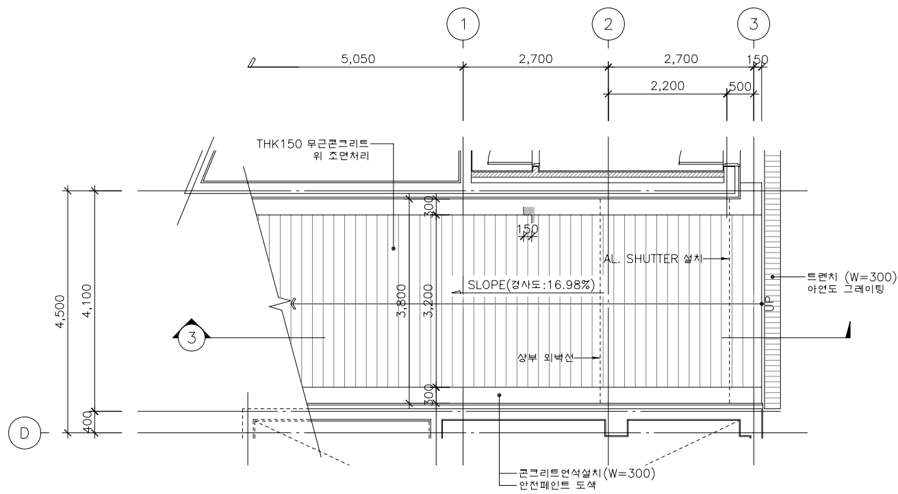
1 지상층 경사로 평면도 축척 : 1/100
