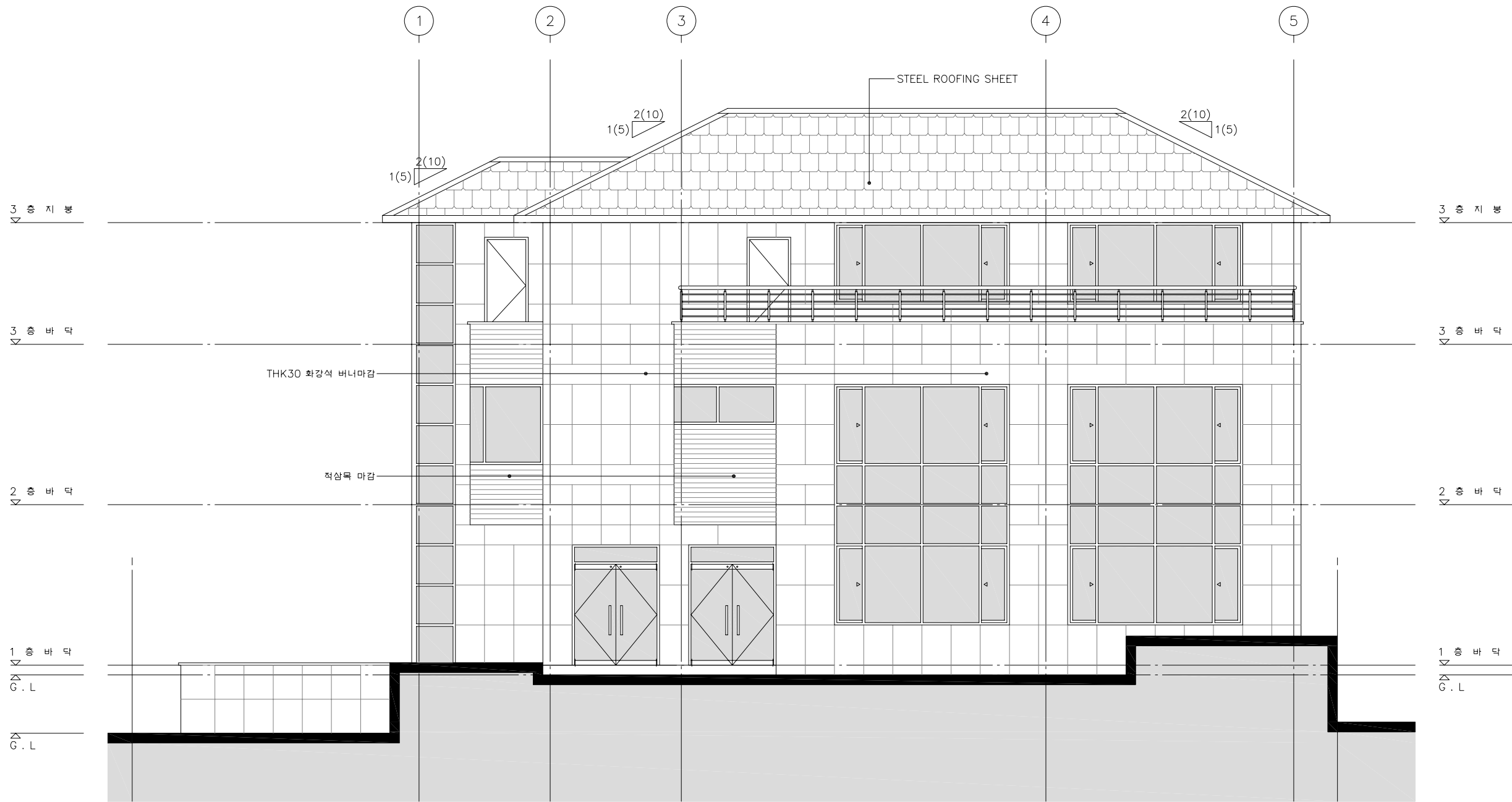
1 정면도 축척 : 1/100
