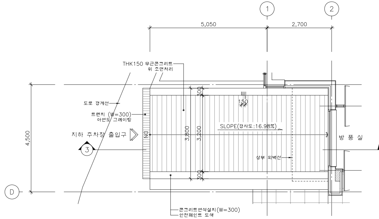
2 지상층 경사로 평면도 축척 : 1/100
