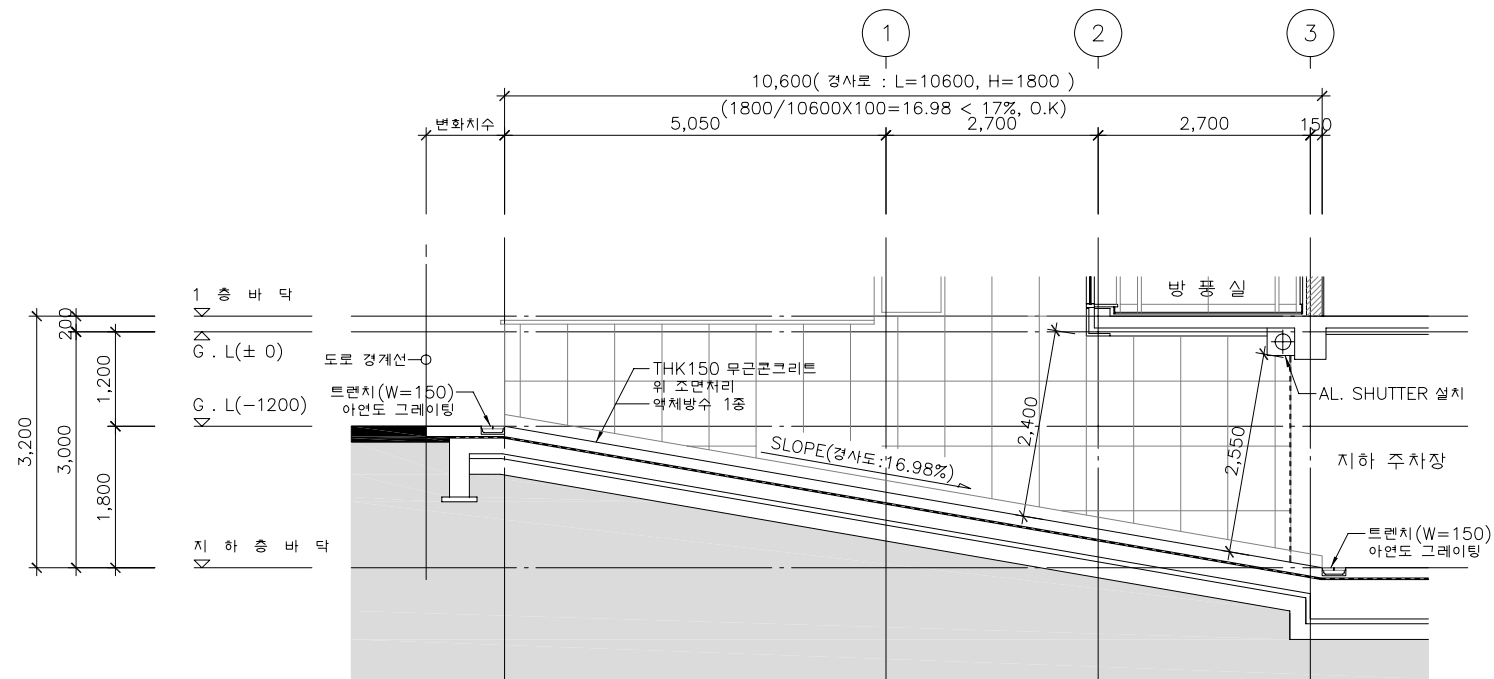
3 경사로 단면도 축척 : 1/100
