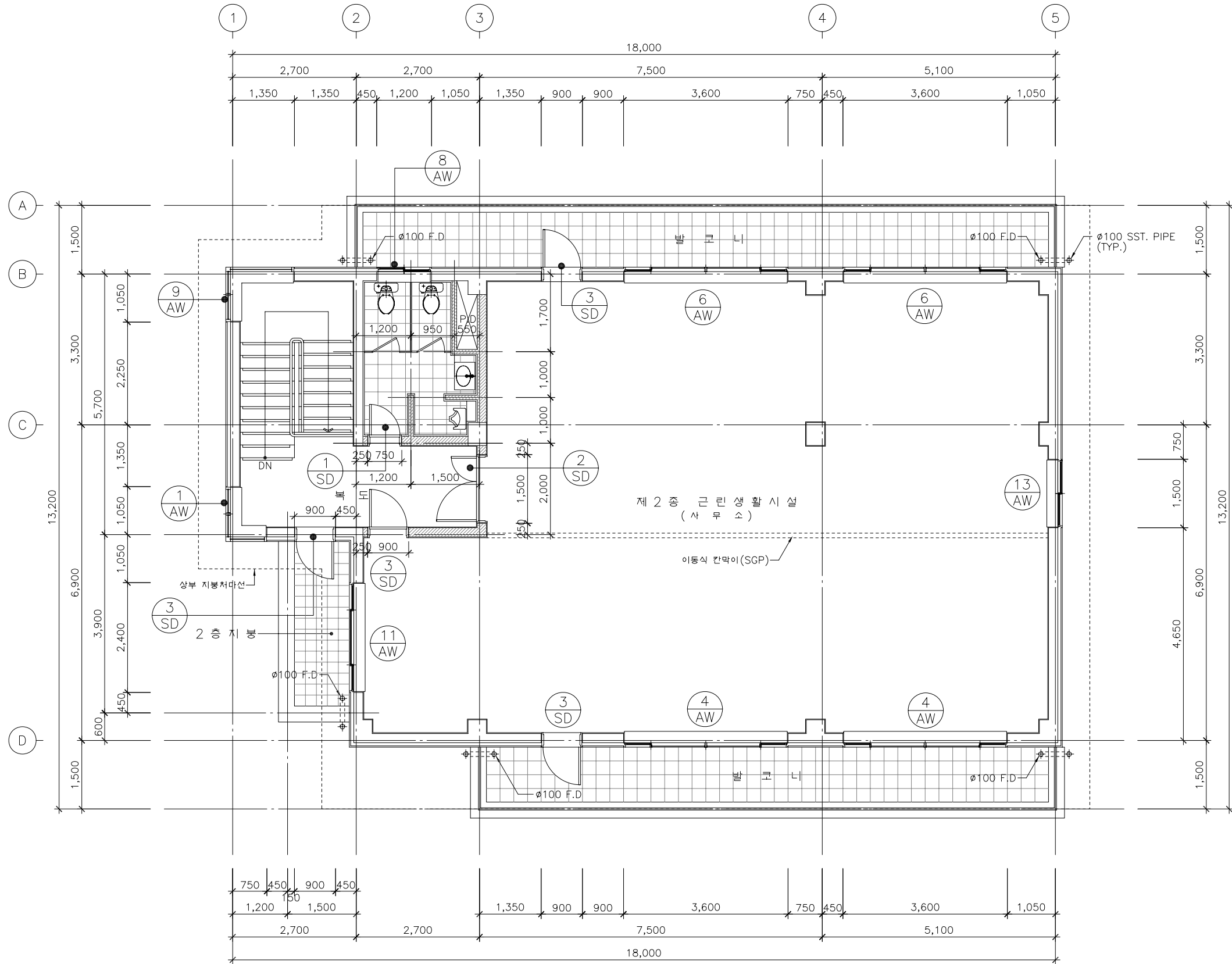
1 3층 평면도 축척 : 1/100
