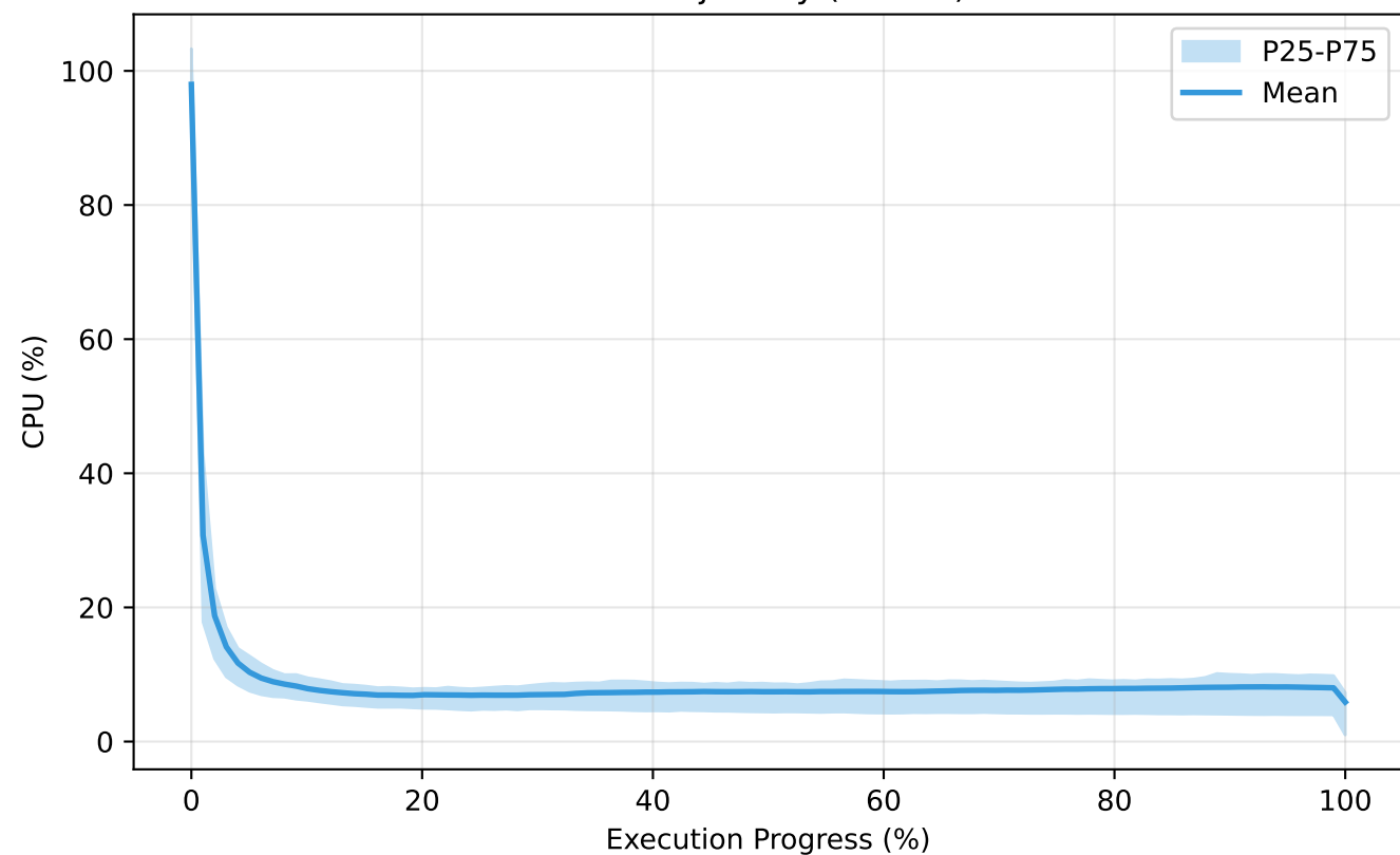
CPU Trajectory (n=111)
