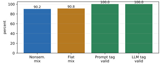
图 2: 当前机制结果。图由 docs/visexp/paper/make_figures.py 从 .agentsight/agentflame/latest/agentflame.json 重新生成; 它反映 Rust full-run 输出, 而不是旧的 Python sampled-run artifact。
