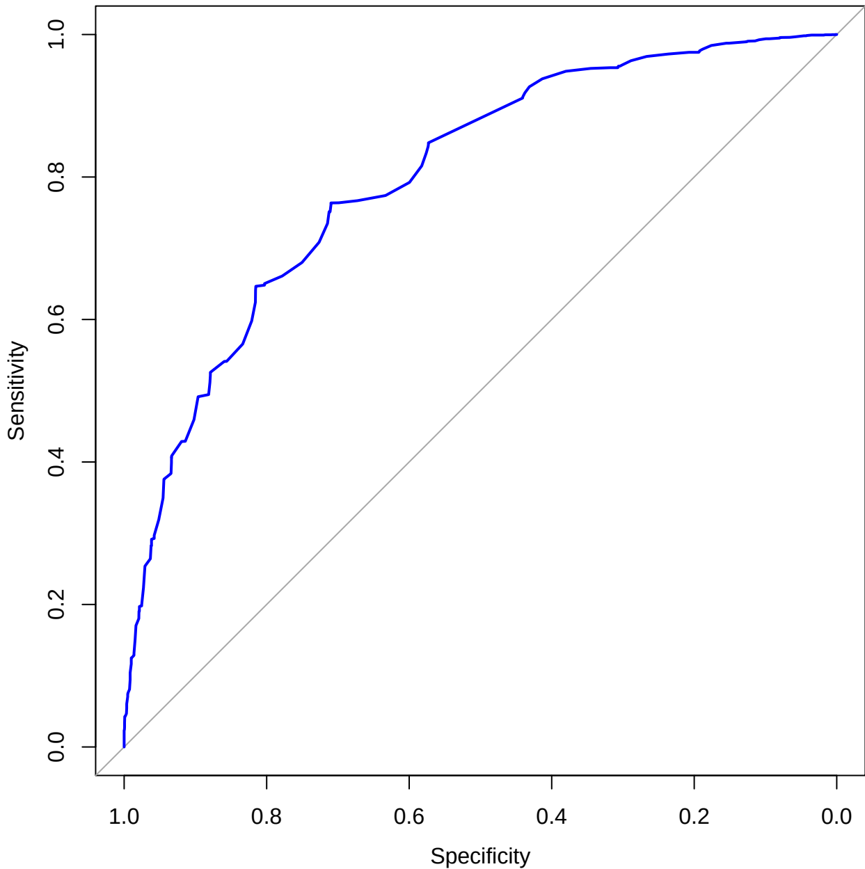
ROC Curve: Binomial CDS Logic
