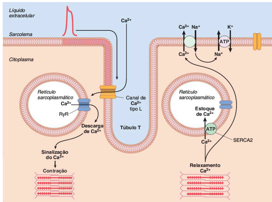
Fig. 4 Acoplamento excitação-contrção e relaxamento. À esquerda, a entrada de \text{Ca}^{2+} pelos canais tipo L dispara a liberação pelo RyR; à direita, a recaptção pela SERCA2 e a saída pelo trocador \text{Na}^+/\text{Ca}^{2+} . (Guyton & Hall, Fig. 9.7)
