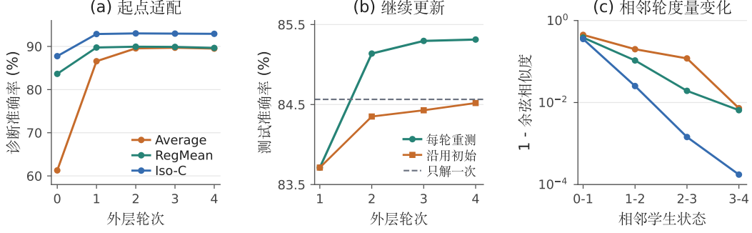
图 1: 当前方法的起点适配、继续修正与度量变化。ViT-B/32, 八任务, seed 0. (a) Average, RegMean, Iso-C 起点在同一独立诊断集上的准确率. (b) Average 的完整测试准确率. 每轮重测: 更新后重新估计 A, G ; 沿用初始: 与前者共享第一轮后固定初始统计. 两支都继续求解与选步. 虚线只做一次共轭梯度, 内层加长至 400 步. (c) 相邻两轮用于求解的 M = G \otimes A 相差多少: 同一批图像上重测并按求解规则处理 A, G , 再对层/任务取 1 减余弦的中位数; 越小表示该度量方向越接近. 纵轴对数尺度, 颜色同 (a). (a) 与 (b) 用不同分割; (c) 固定统计图像. 定义见附录 A. 三面板均使用本文的 KL 修正统计.
