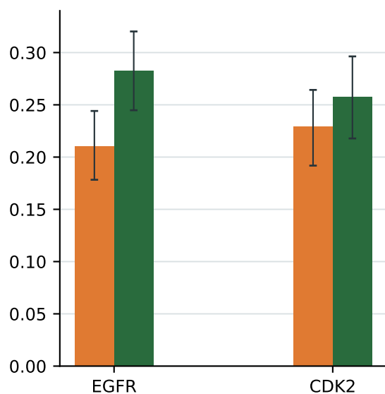
BEDROC
