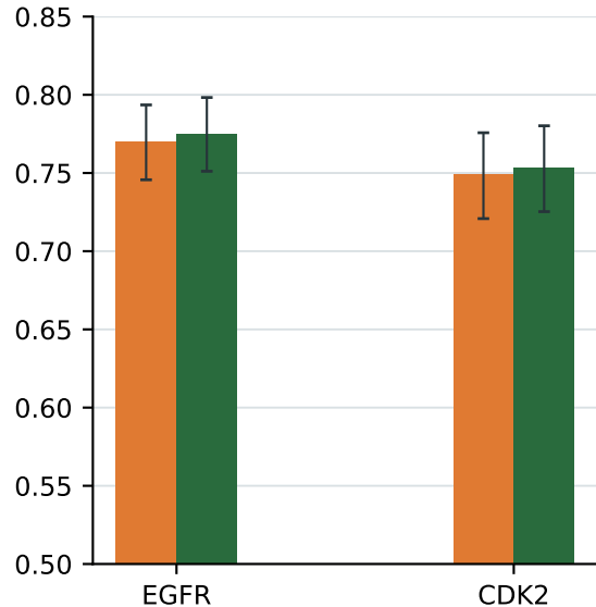
ROC-AUC
