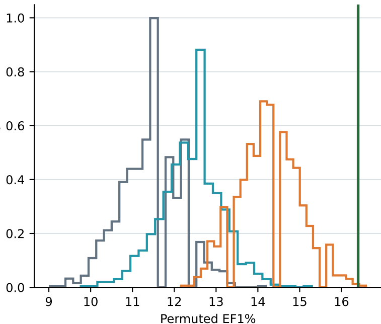
EGFR
