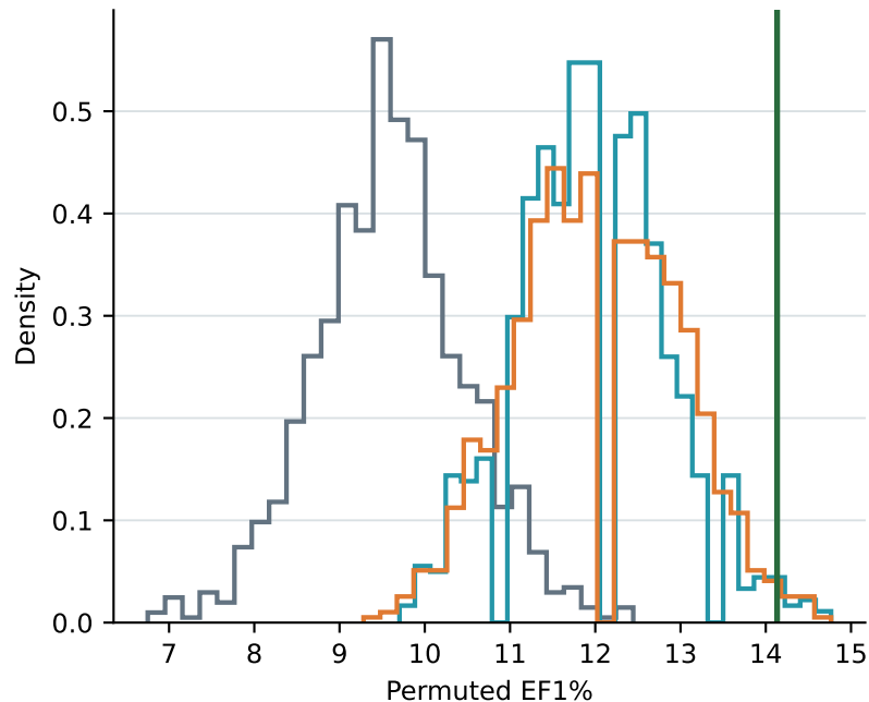
CDK2
