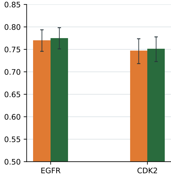
ROC-AUC
