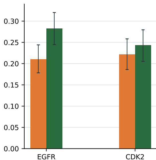
BEDROC
