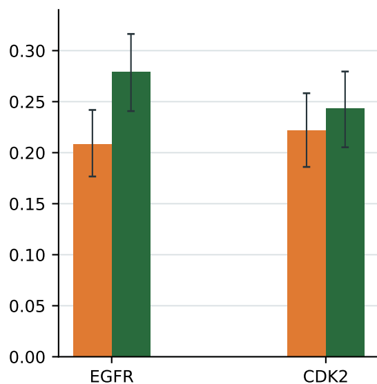
BEDROC
