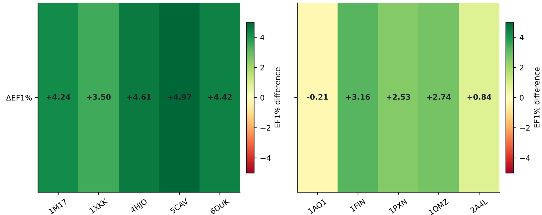
EGFR
