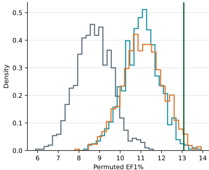
CDK2
