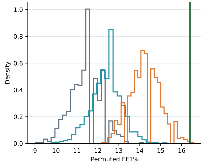
EGFR
