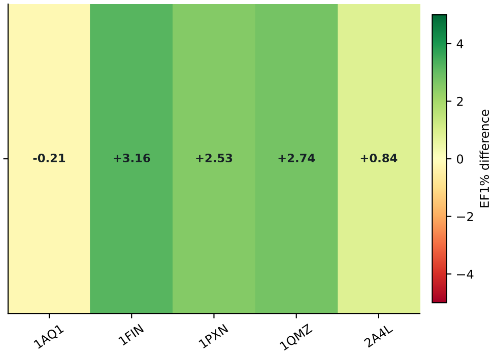
CDK2
