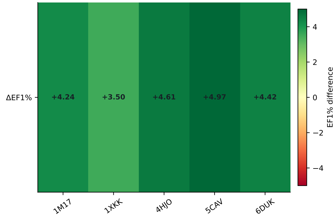
EGFR
