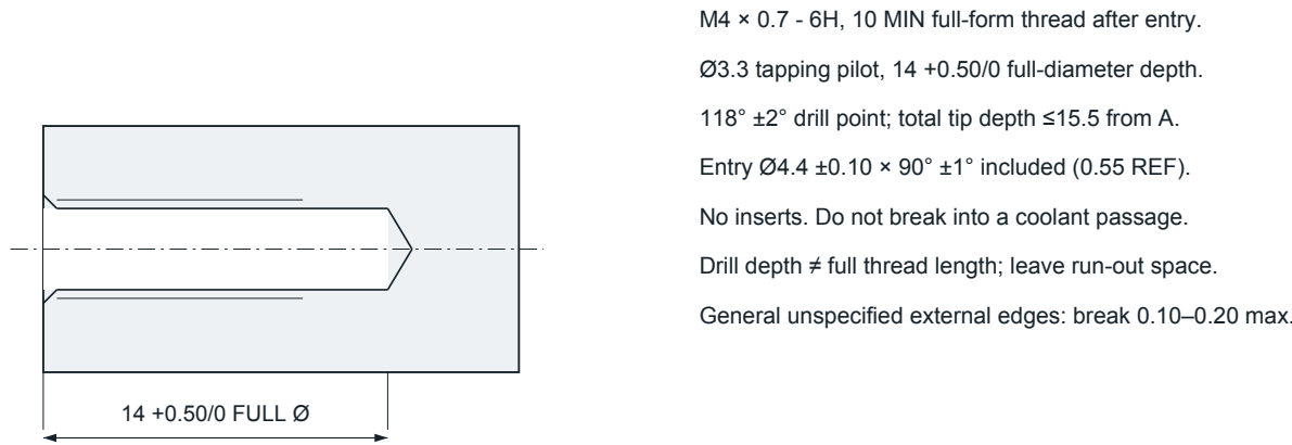
DETAIL C — M4 × 0.7 - 6H (6 places), 3:1
