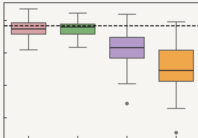
MOGP
