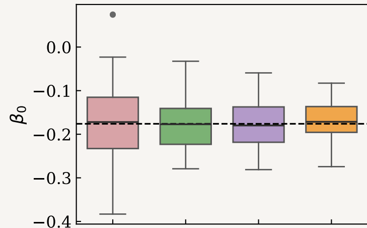
MOOGP
