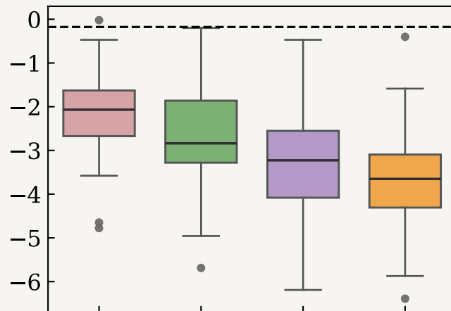
MOGP
