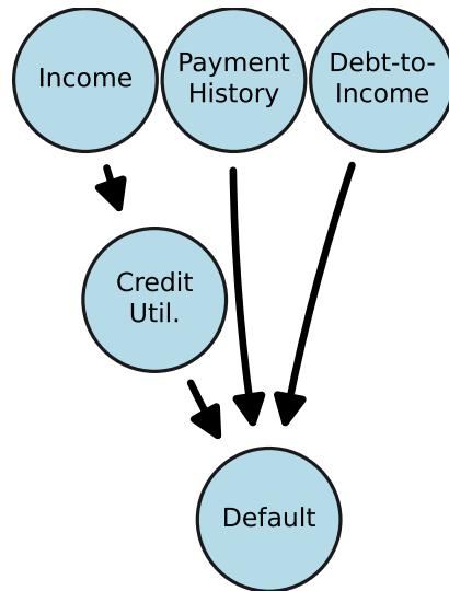
Neuron DAG
