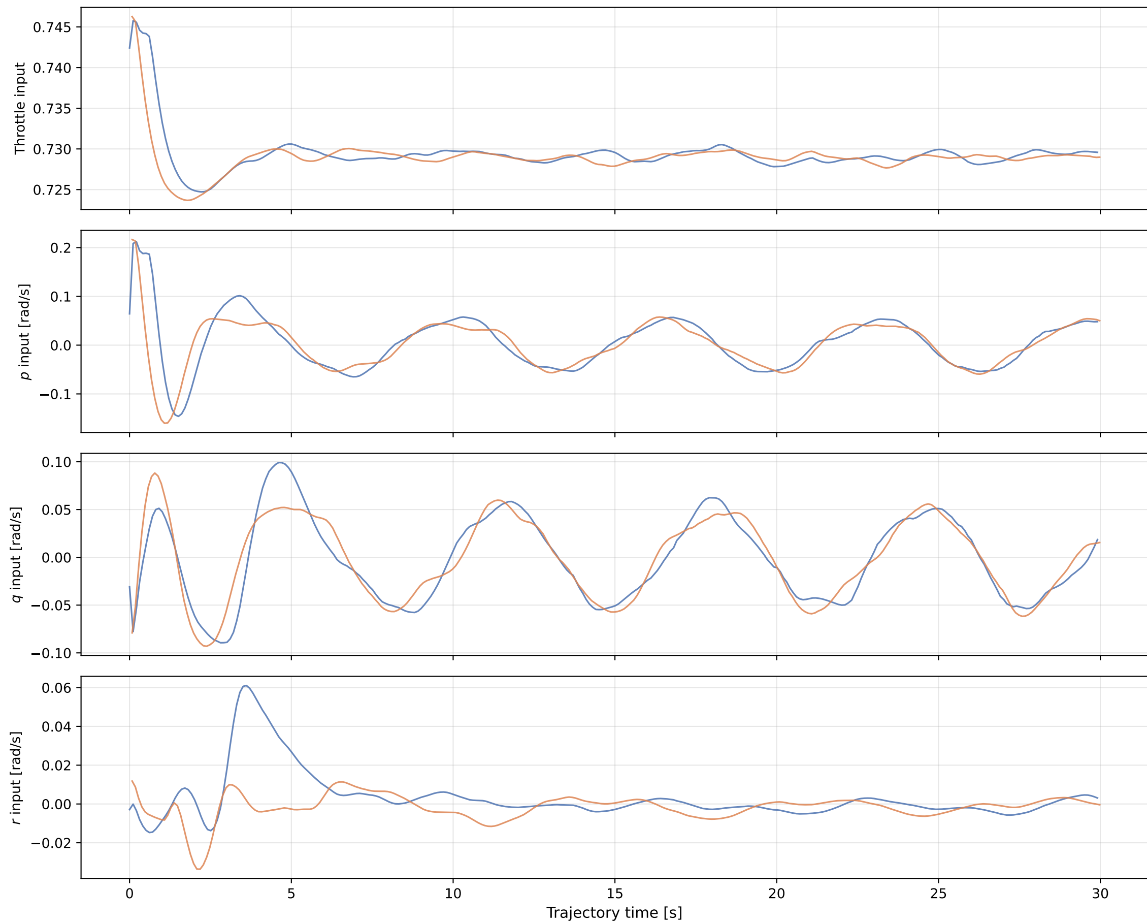
Control Inputs — Circle Horz 2x
