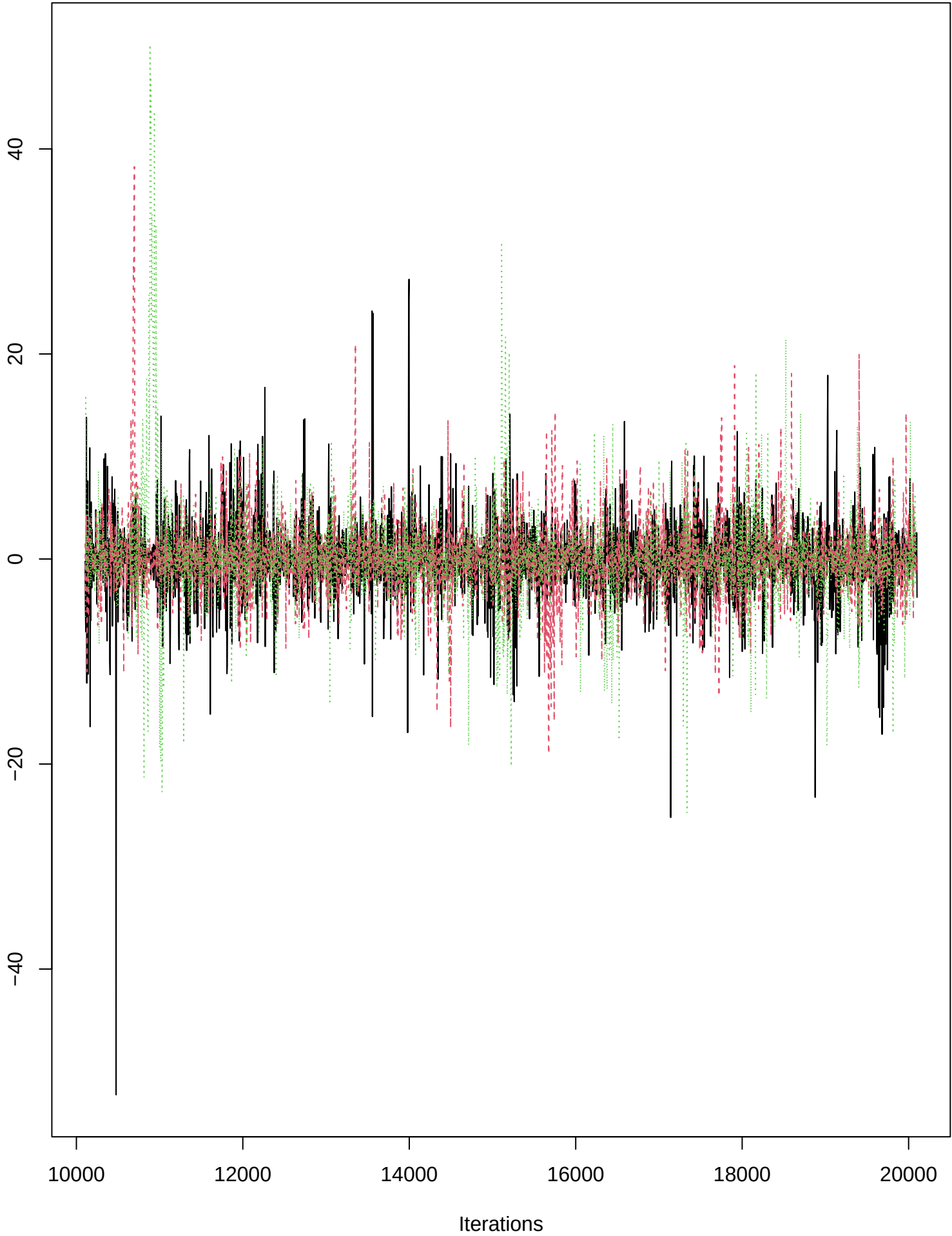
Trace of beta_mon_egg[11]
