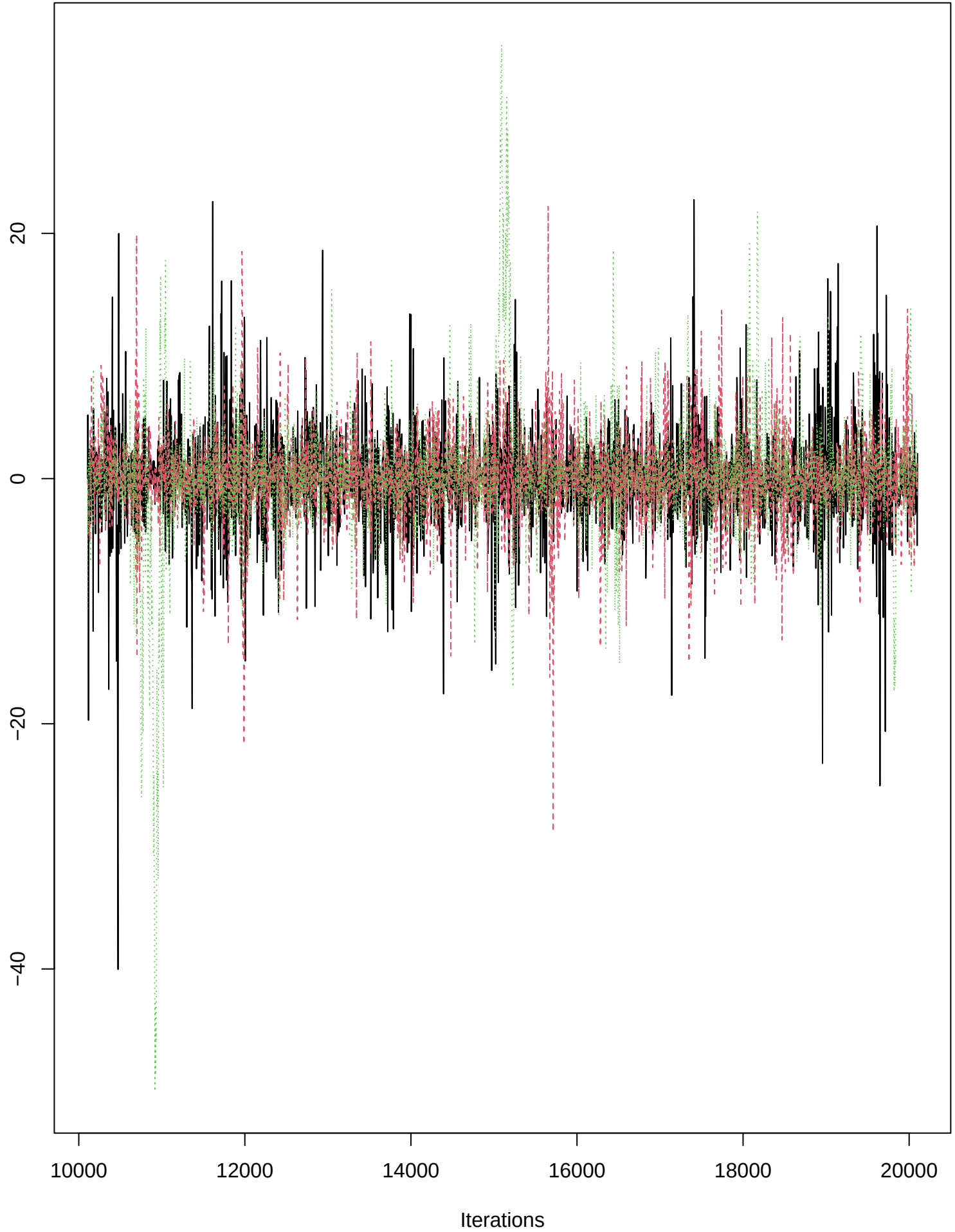
Trace of beta_mon_egg[12]
