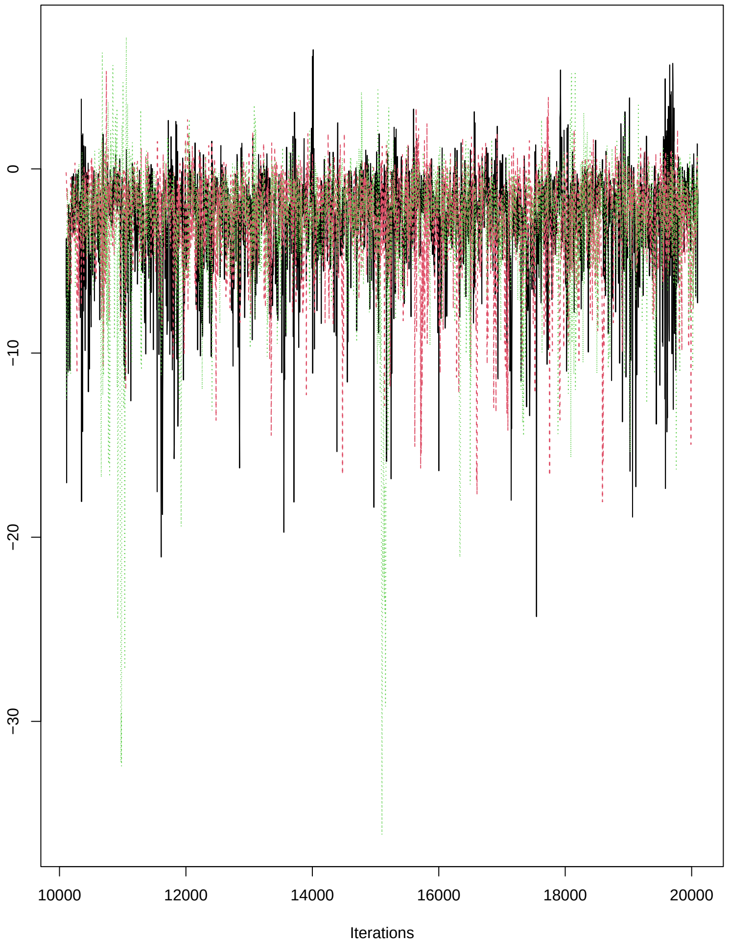
Trace of beta_mon_egg[1]
