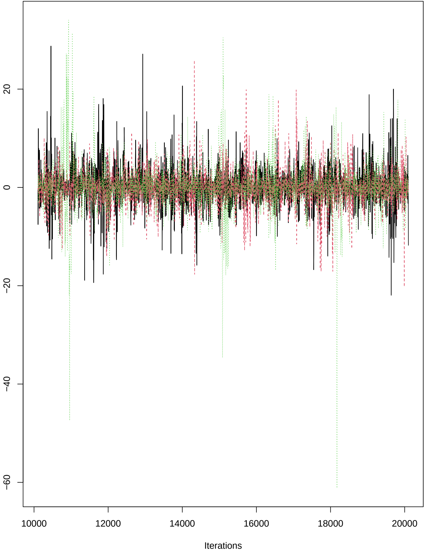
Trace of beta_mon_egg[10]
