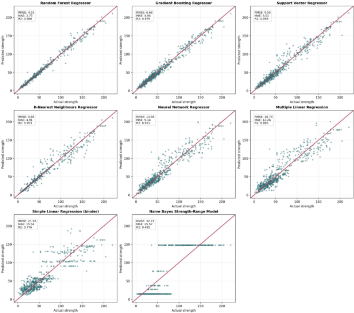
Actual vs Predicted Concrete Strength
