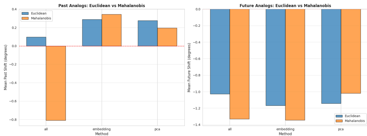
Fig. 4. – Translation latitudinale moyenne par méthode et métrique de distance. Gauche : Période passée (1970). Droite : Période future (2050, moyenne des 3 scénarios SSP).
