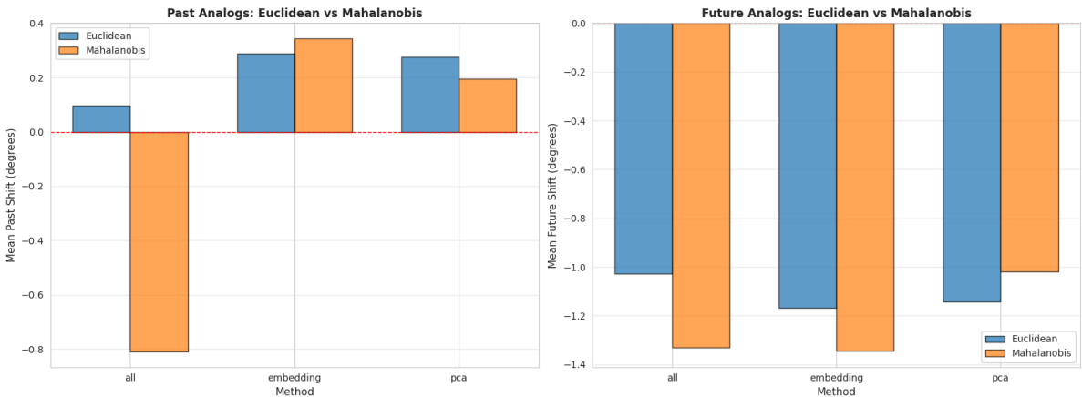
Fig. 4. – Translation latitudinale moyenne par méthode et métrique de distance. Gauche : Période passée (1940-1970). Droite : Période future (2021-2050, moyenne des 3 scénarios SSP).
