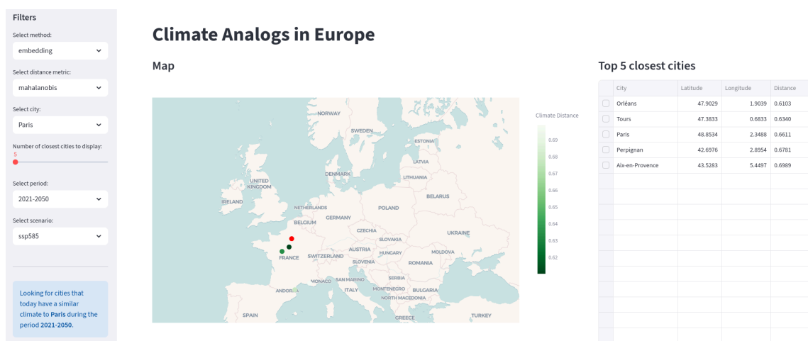
Fig. 3. – Application interactive montrant les analogues climatiques de Paris pour la période 2021-2050 (scénario SSP585, méthode Embeddings, distance de Mahalanobis). Les 5 villes les plus proches sont : Orléans, Tours, Paris, Perpignan et Aix-en-Provence.
