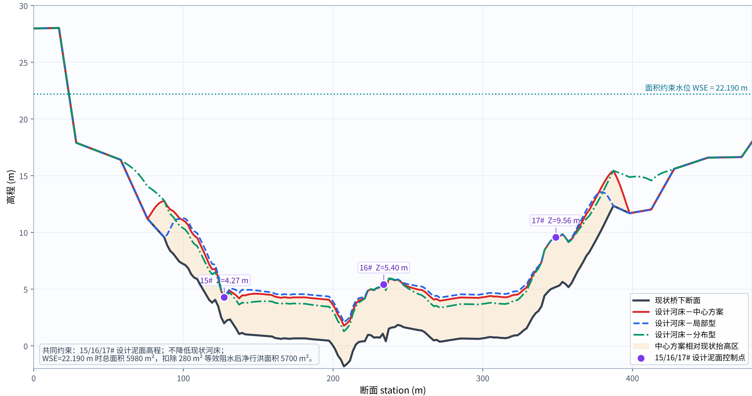
桥下断面：现状河床与三种设计河床重建方案
