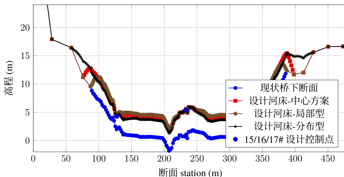
图 6: 现状桥下断面与三种受约束设计河床重建
