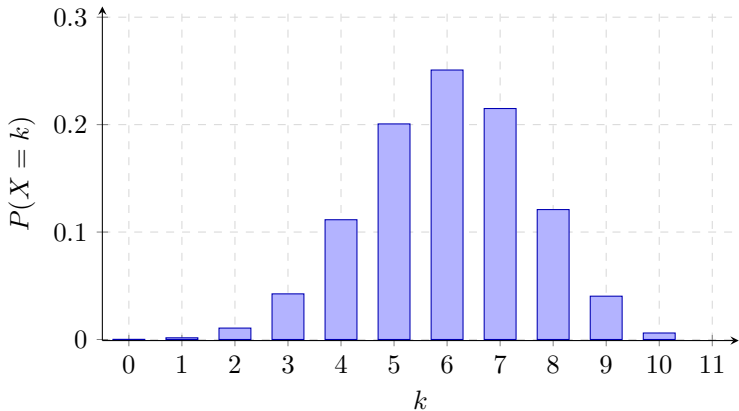
Binomial distribution \text{Binom}(10, 0.6)
