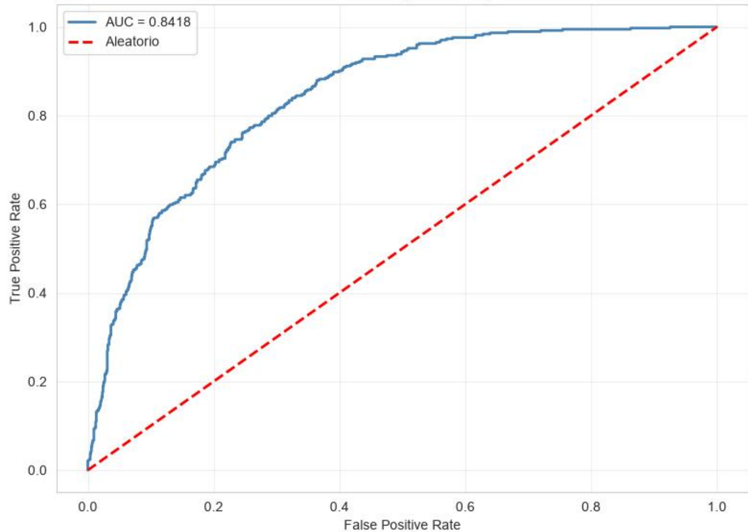
Curva ROC — Regresión Logística
