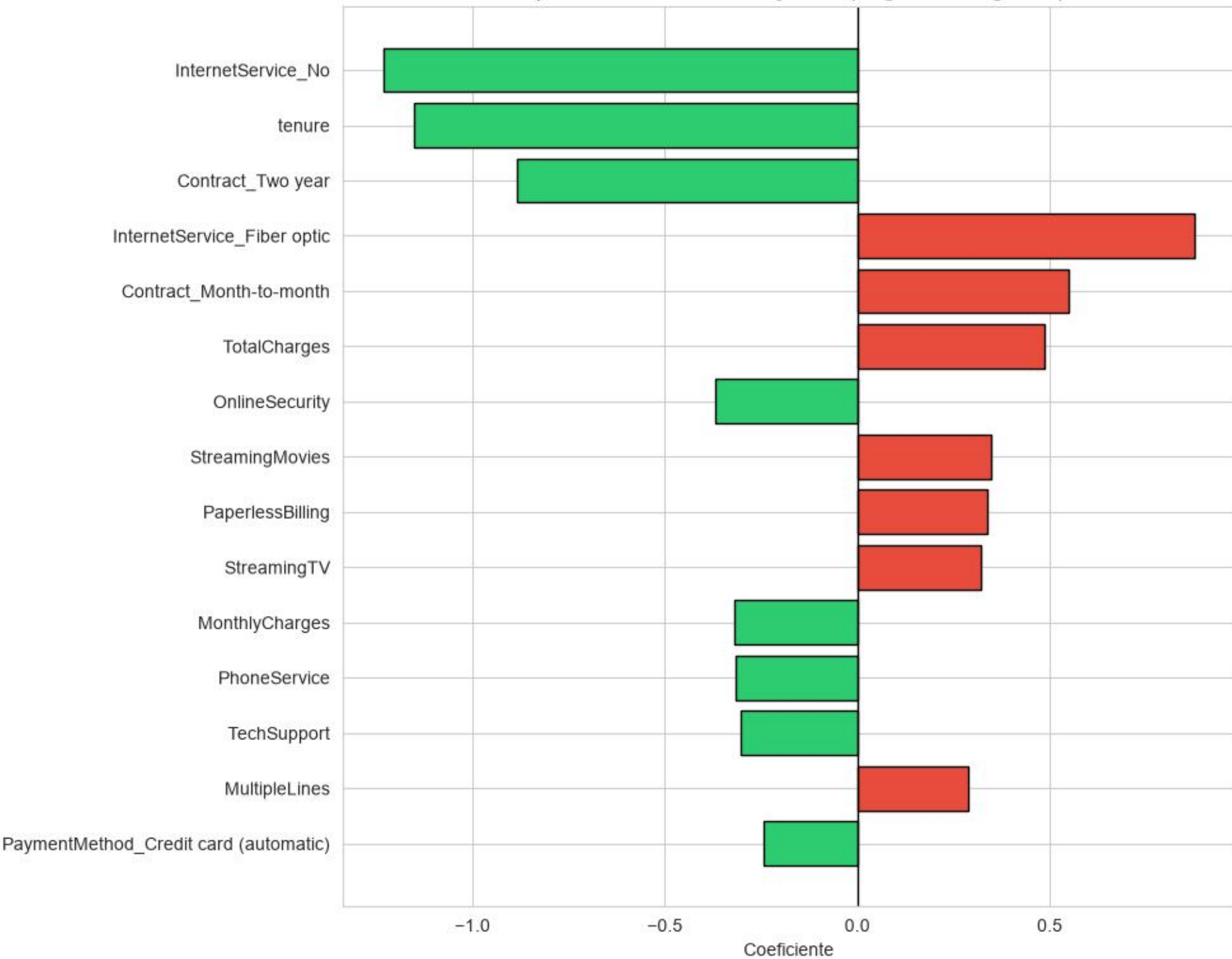
Top 15 variables más influyentes (Regresión Logística)
