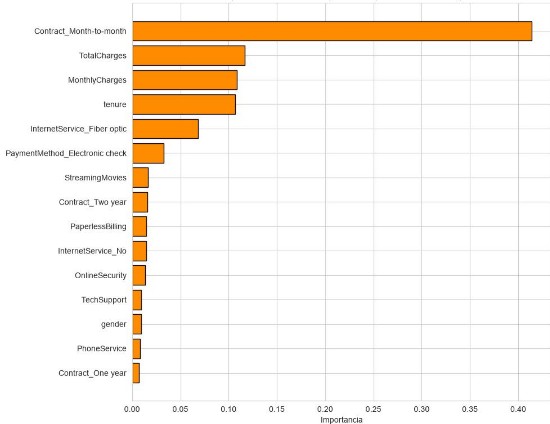
Top 15 variables más importantes (Gradient Boosting)
