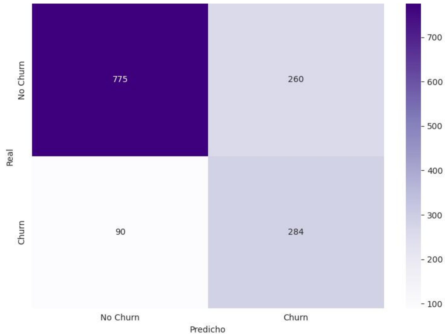
Matriz de Confusión — Red Neuronal
