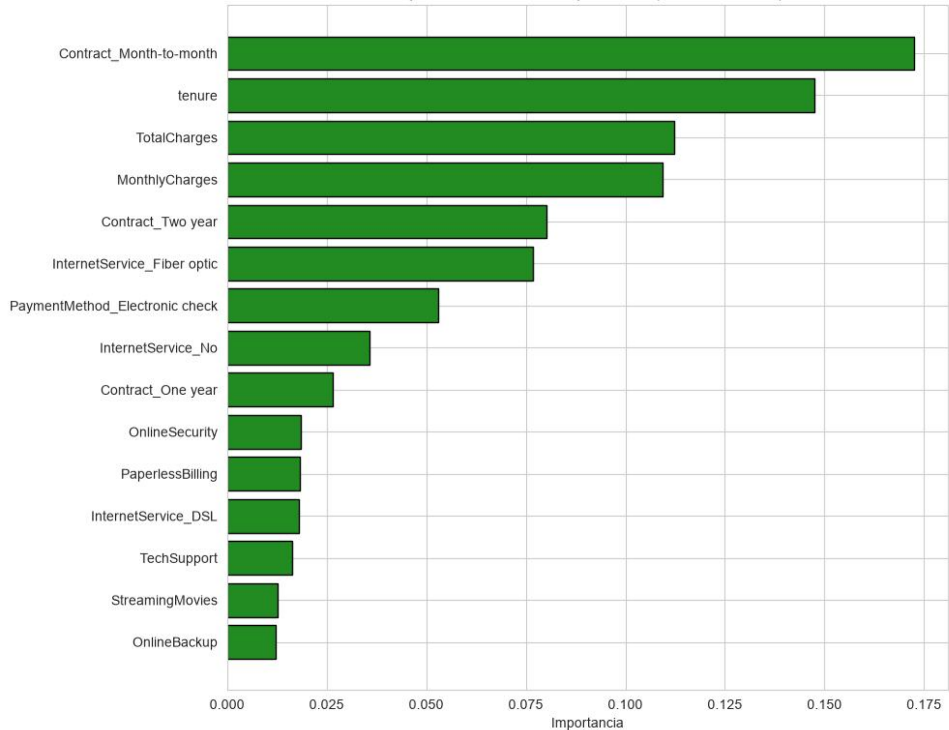
Top 15 variables más importantes (Random Forest)
