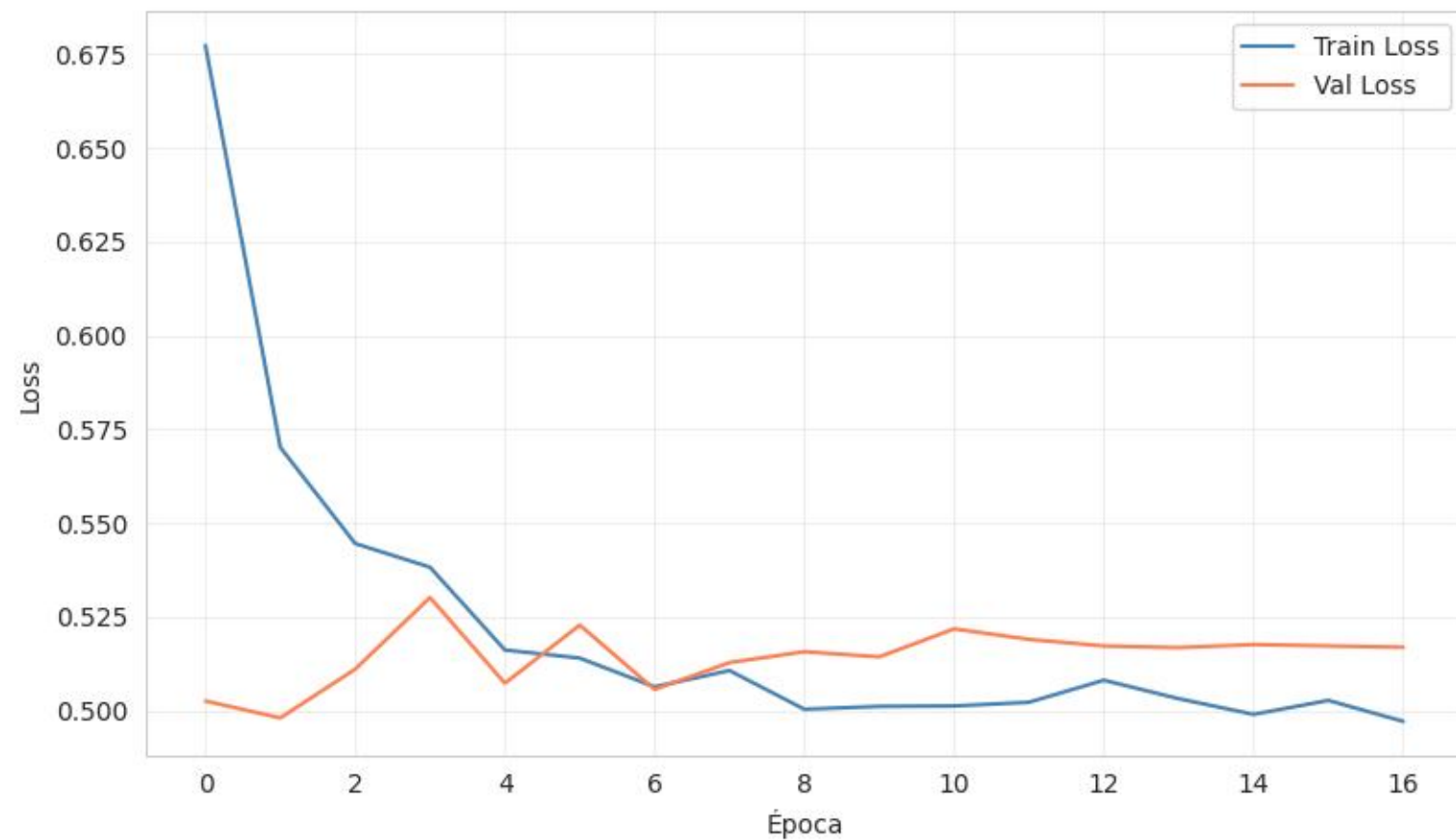
Pérdida durante el entrenamiento
