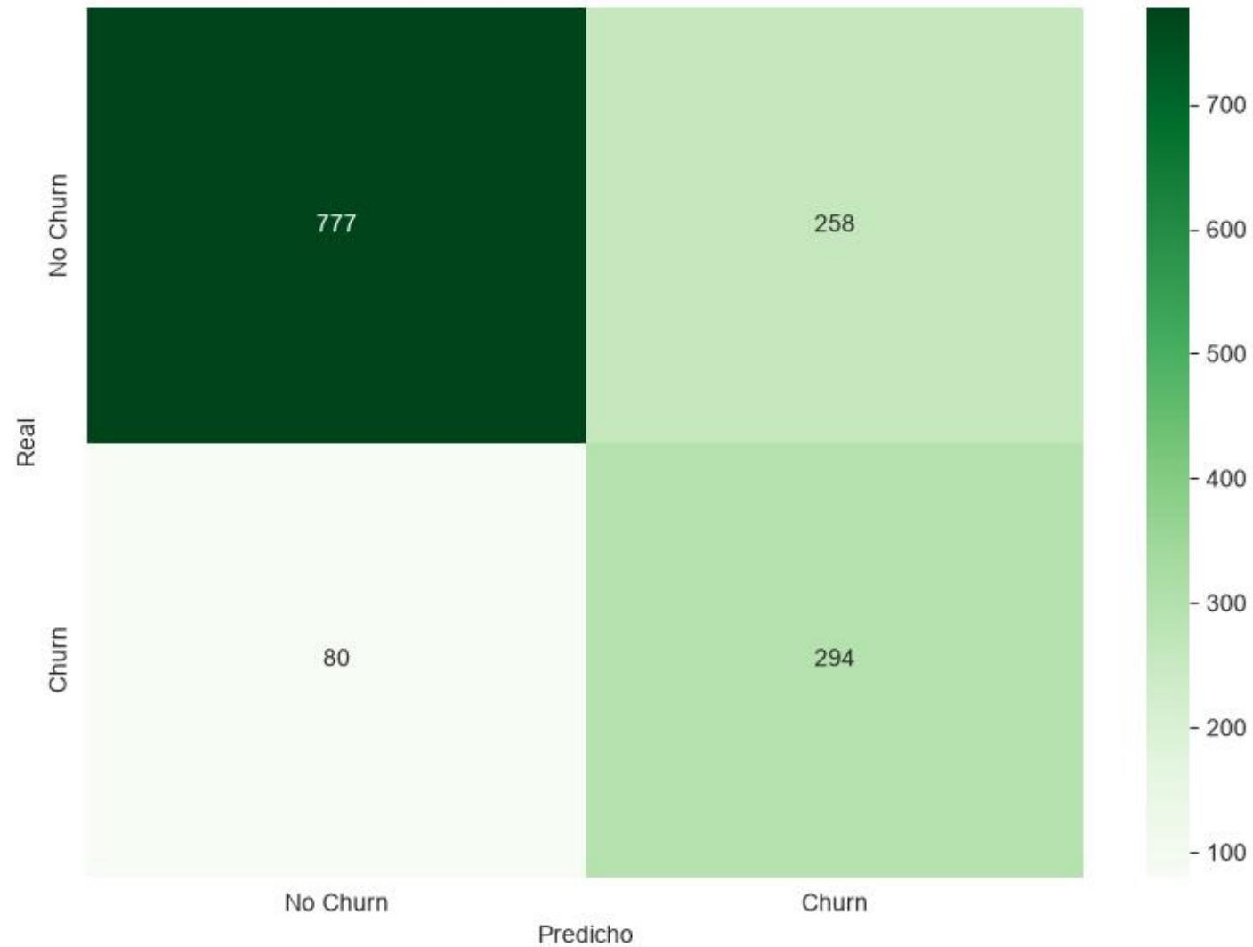
Matriz de Confusión — Random Forest
