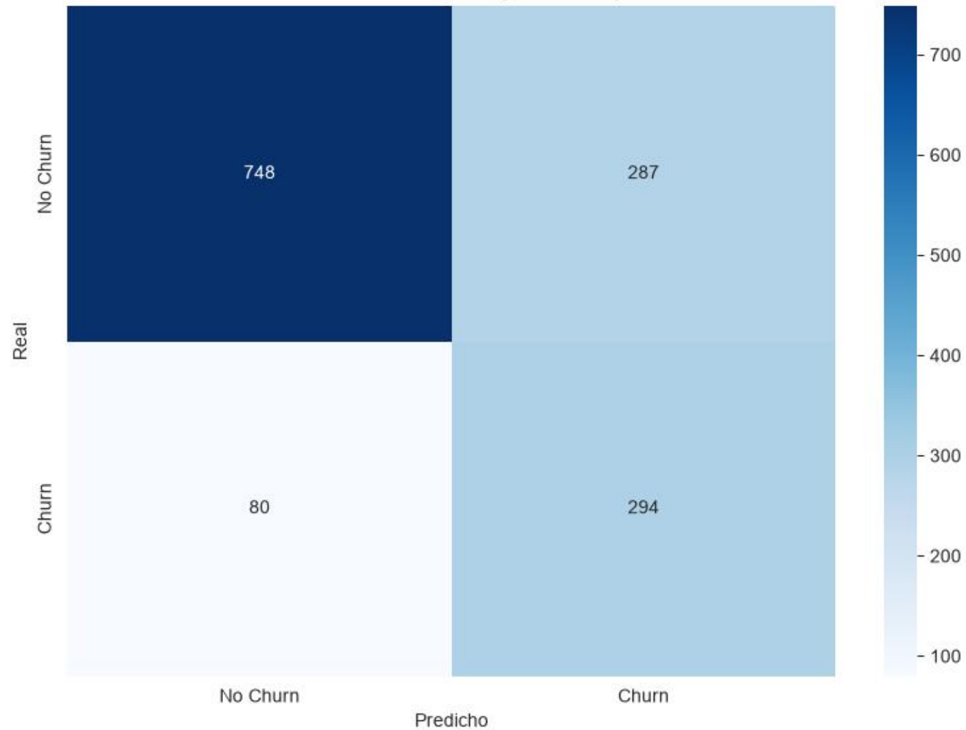
Matriz de Confusión — Regresión Logística
