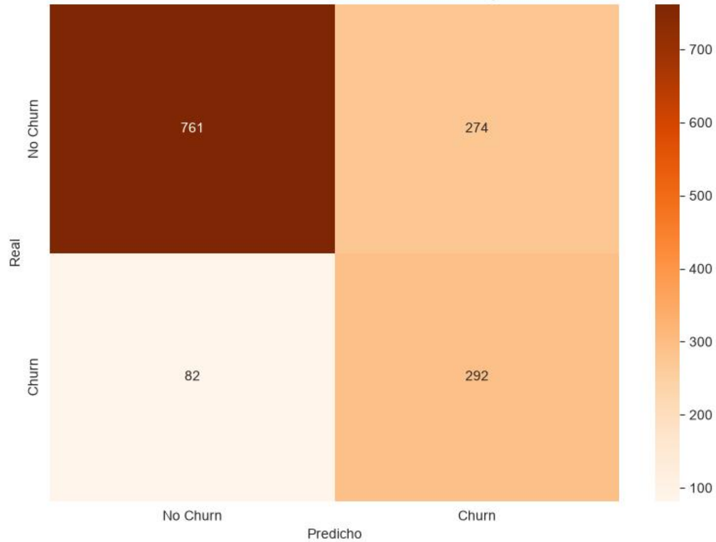
Matriz de Confusión — Gradient Boosting
