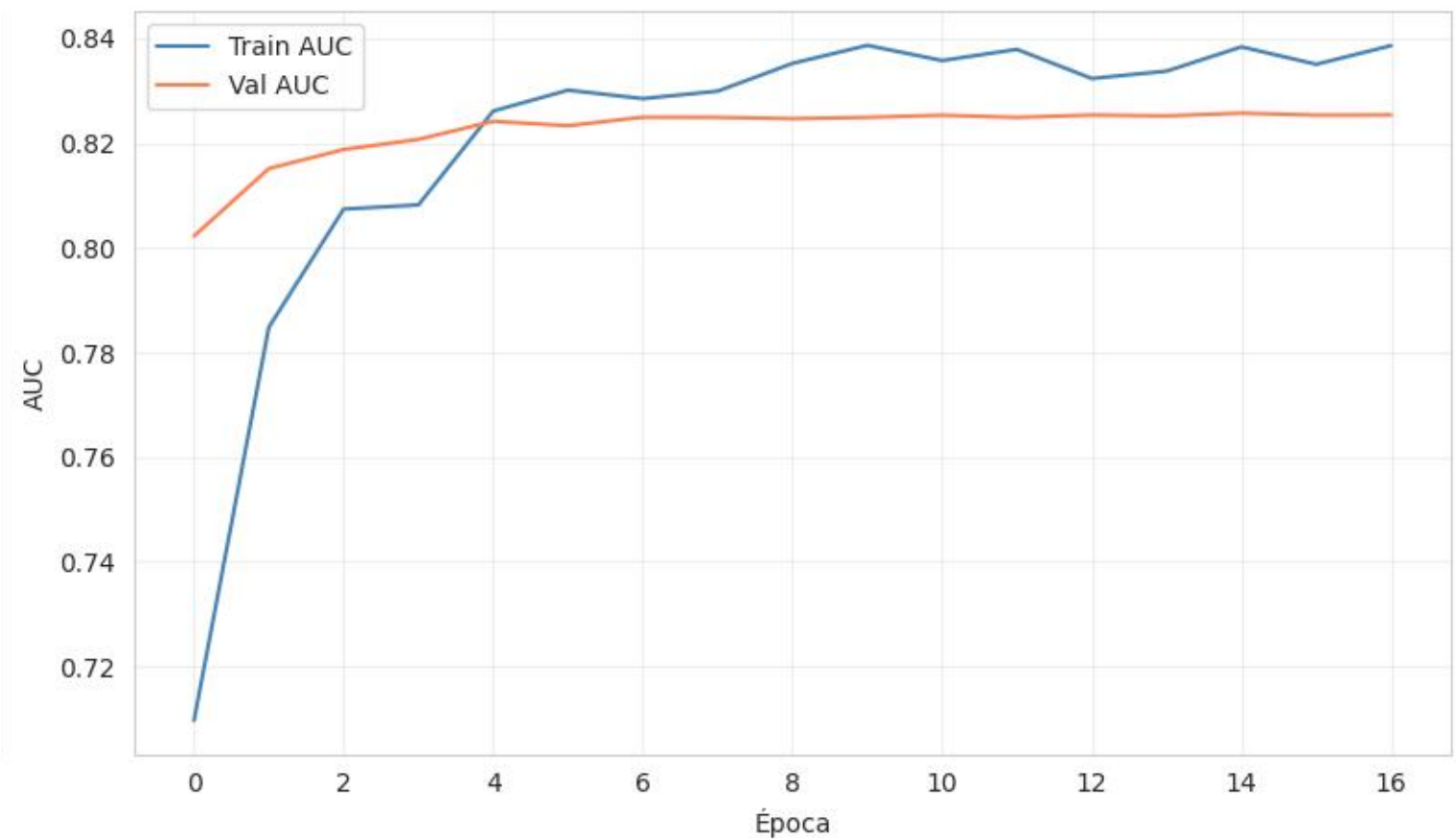
AUC durante el entrenamiento
