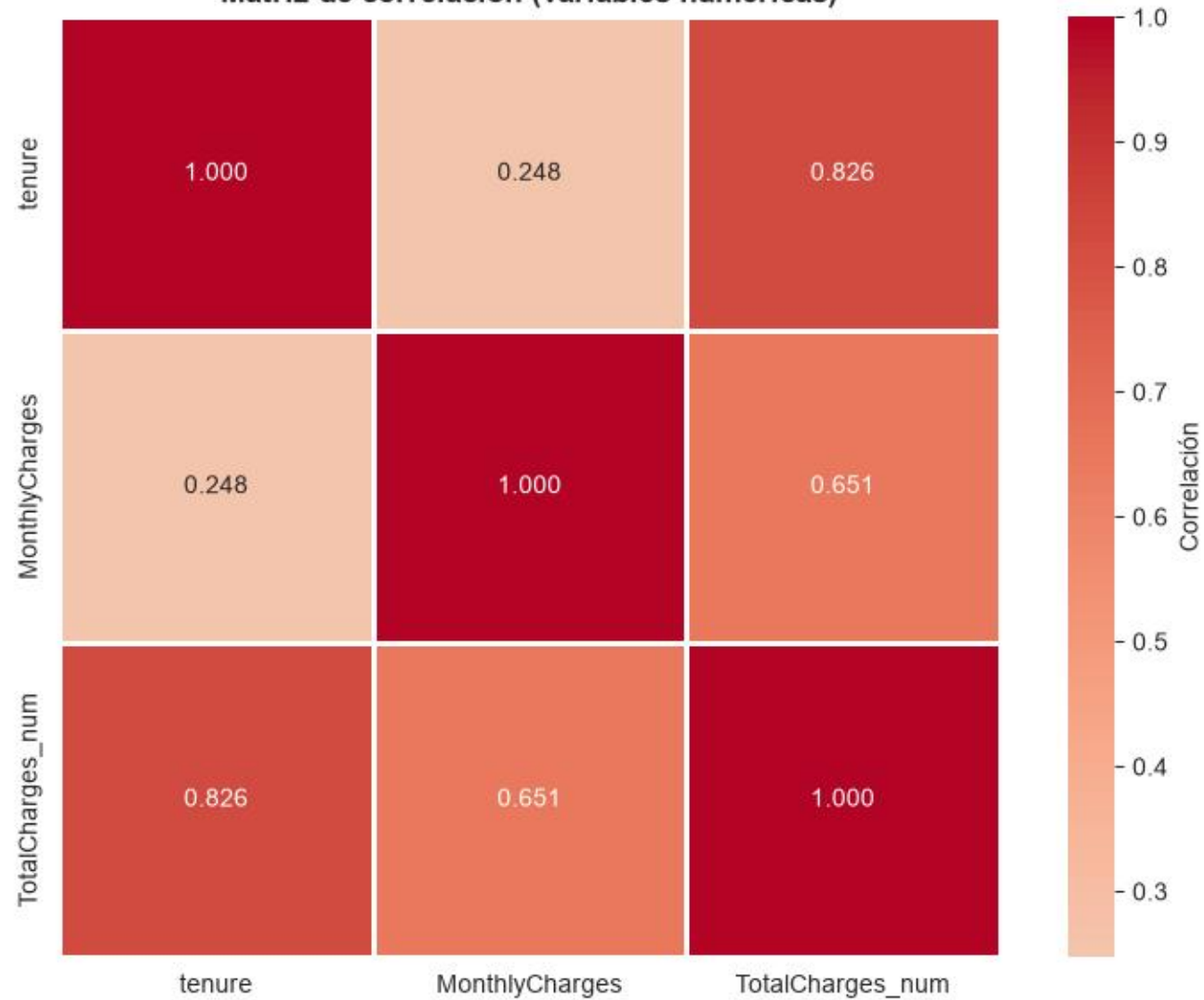
Matriz de correlación (variables numéricas)
