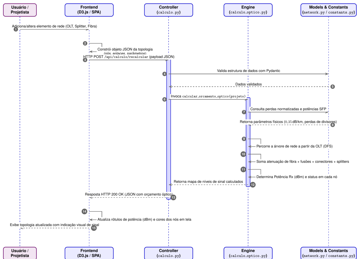
Figura 34 – Diagrama de sequência do recálculo óptico em tempo real
