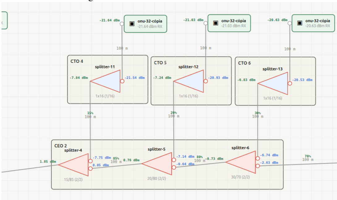
Figura 42 – Bloco 2 do diagrama no PON Planner – CEO-2 e CTOs 4 a 6
