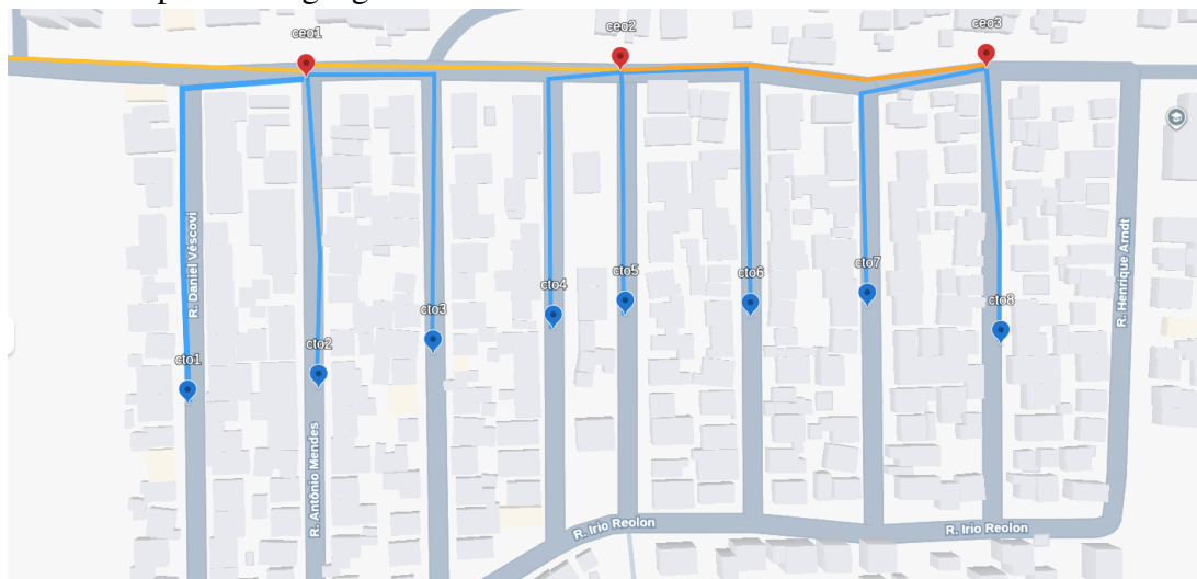
Figura 37 – Mapeamento geográfico da rede GPON em área urbana
