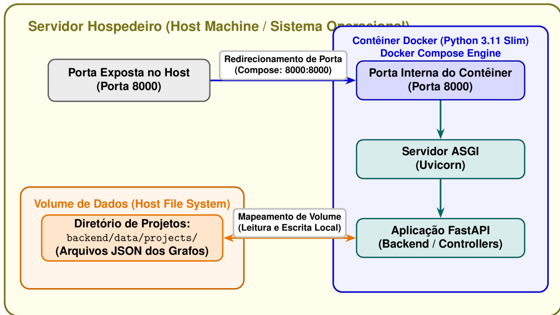
Figura 33 – Diagrama de implantação do sistema containerizado
