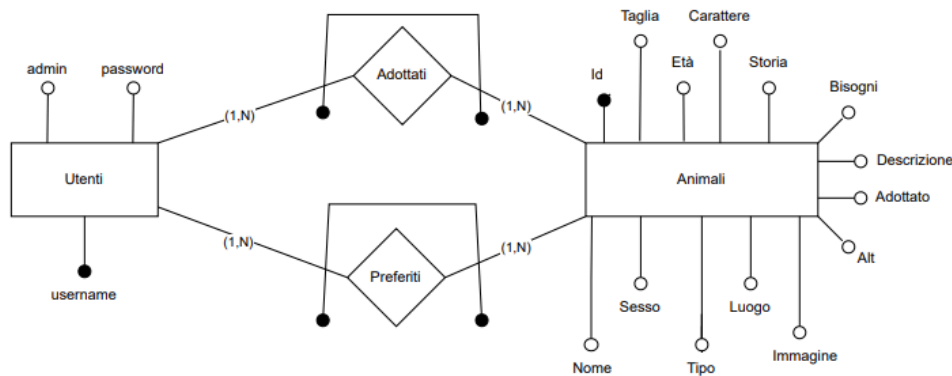
Figura 2: E-R Database
