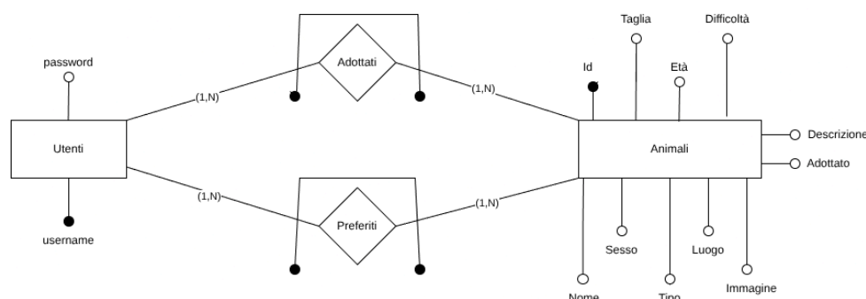
Figura 2: E-R Database
