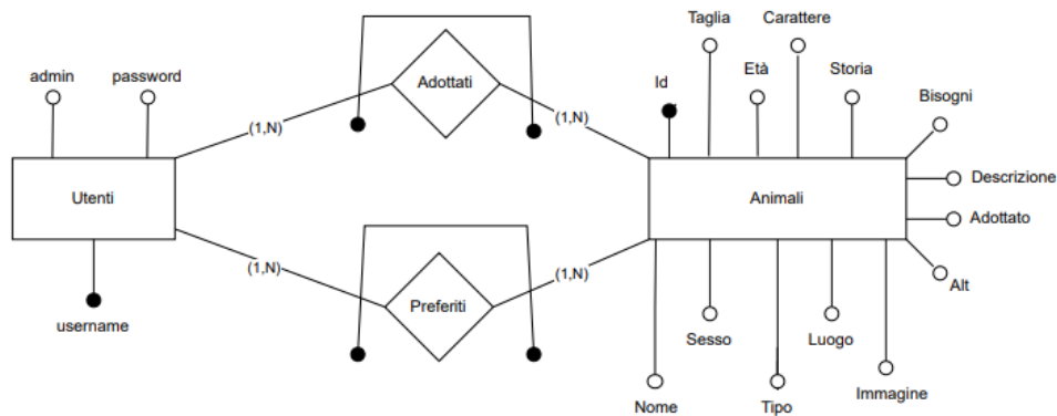
Figura 2: E-R Database
