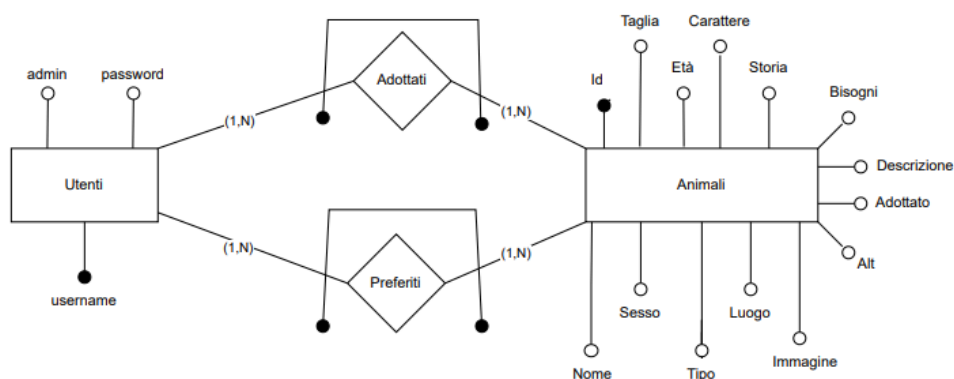
Figura 2: E-R Database
