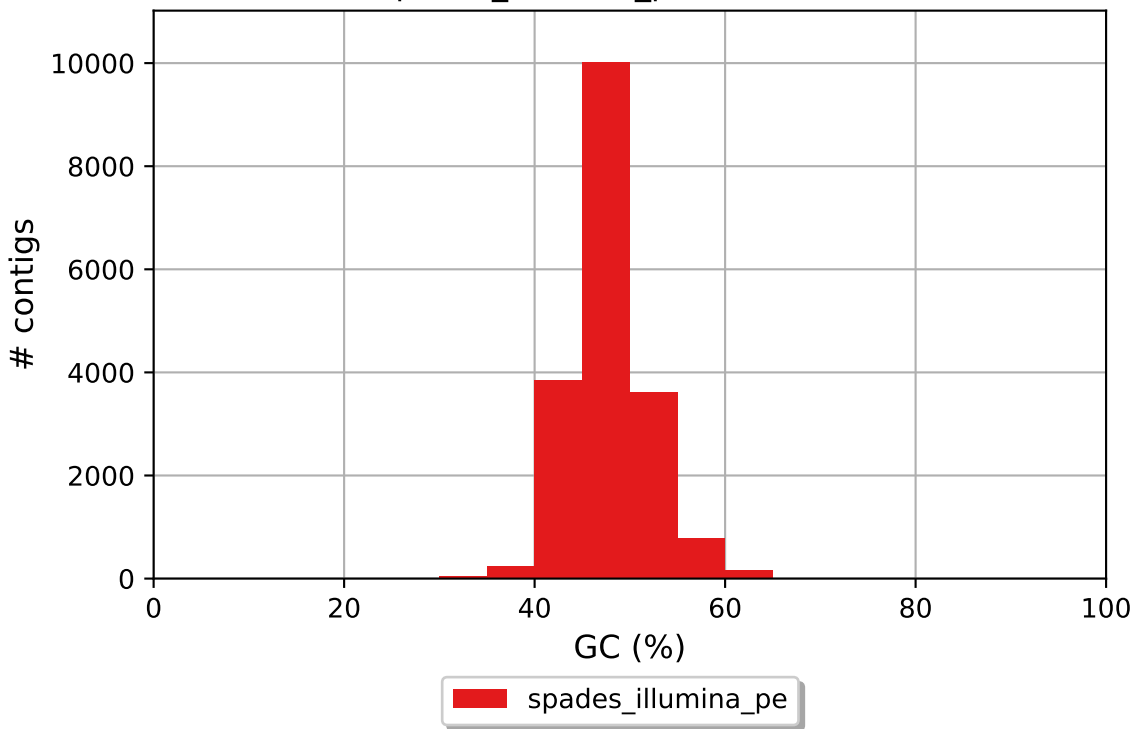
spades_illumina_pe GC content
