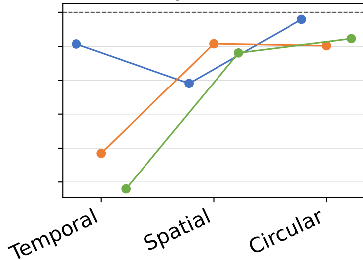
Jeffreys-Dirichlet
