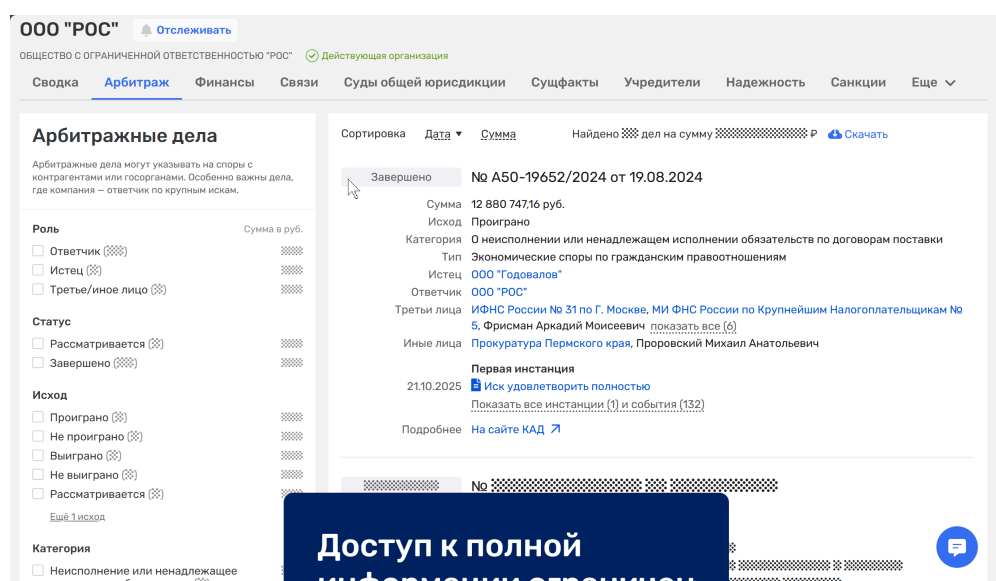
Рис. 17: Пример интерфейса прецедента 8: вкладка «Арбитраж» карточки контрагента — список дел с фильтрацией и ограничение доступа для гостей
