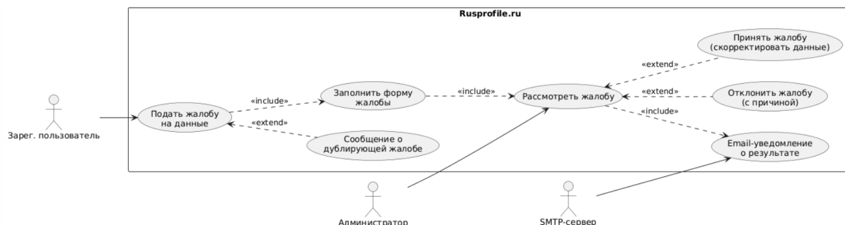
Рис. 24: Диаграмма прецедента 12: Модерация жалоб на данные
