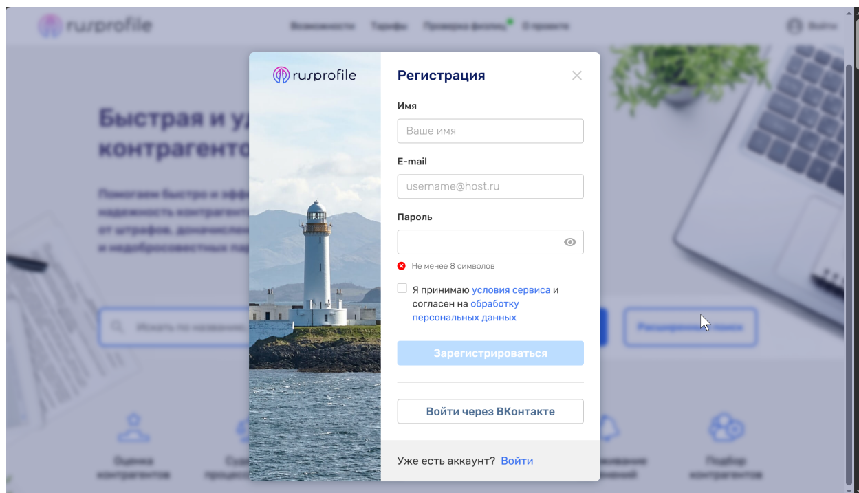
Рис. 9: Пример интерфейса прецедента 4: форма регистрации — поля e-mail и пароль, валидация, вход через OAuth (ВКонтакте)
