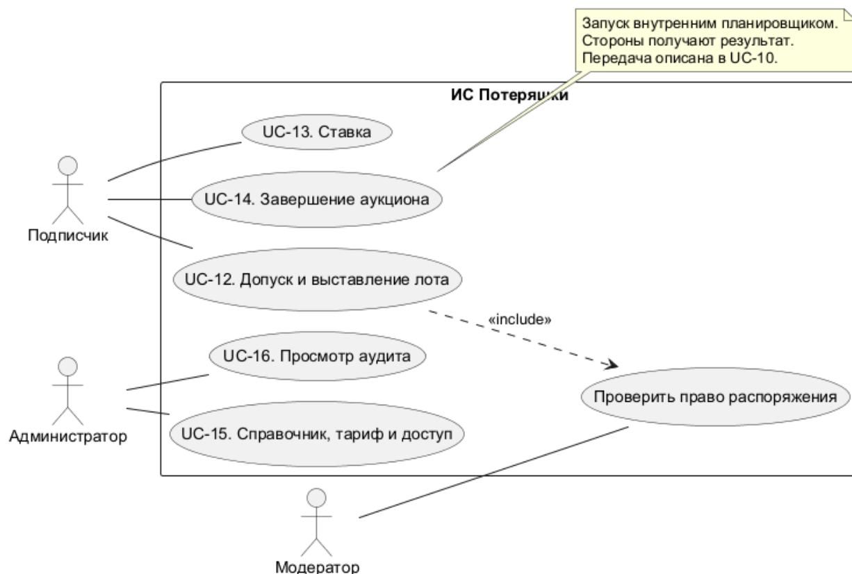
Рисунок 3 — UML-прецеденты аукциона и администрирования
