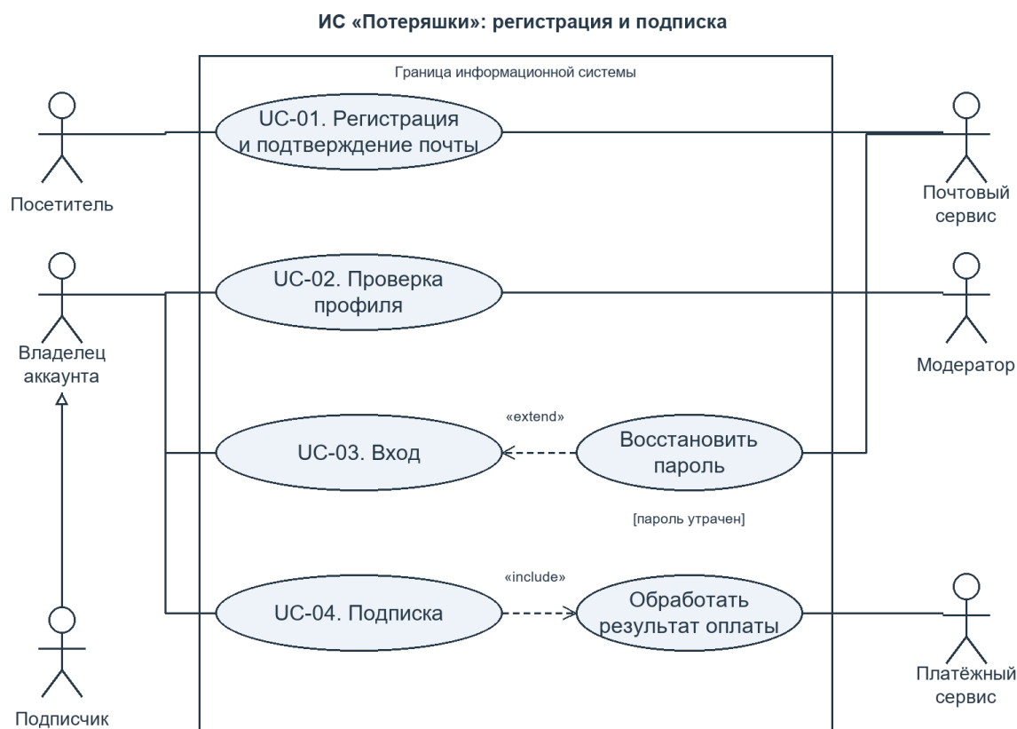
Рисунок 1 — UML-прецеденты регистрации и подписки
