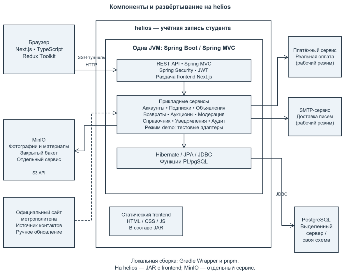
Рисунок 4 — Компоненты и развёртывание на helios
