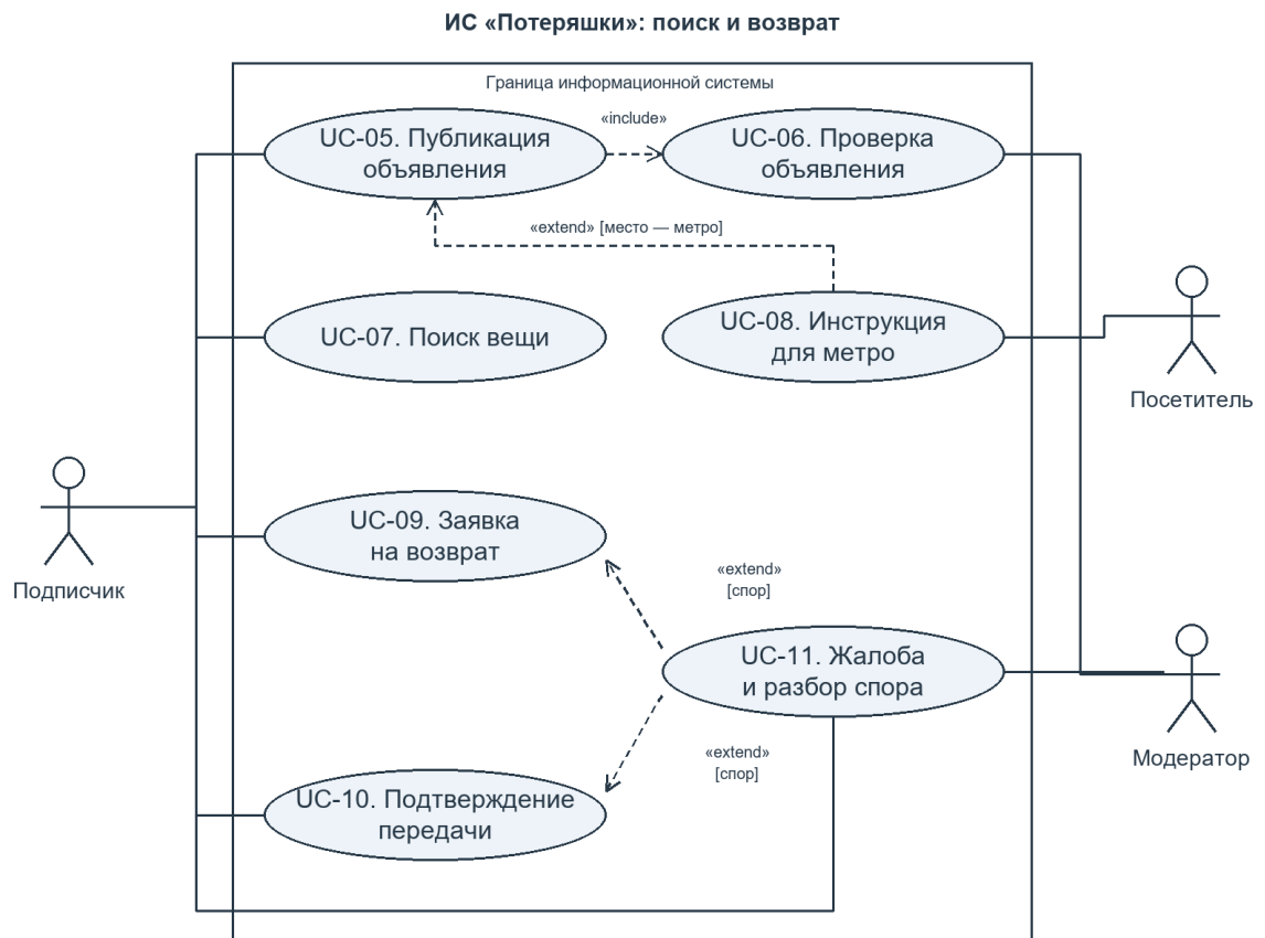
Рисунок 2 — UML-прецеденты поиска и возврата
