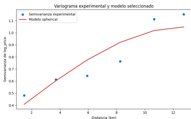
Figura 11. Semivarianza experimental y variograma esférico seleccionado.
