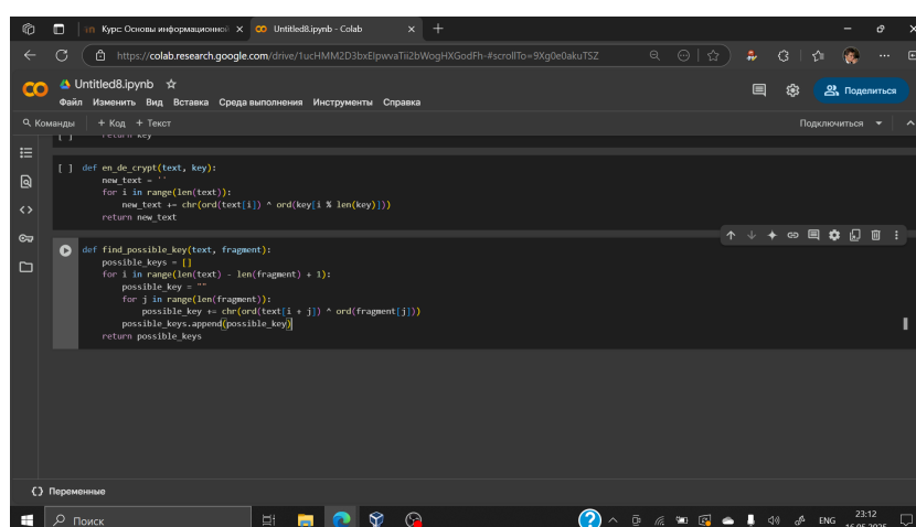
Рис. 4.3: Подбор возможных ключей для фрагмента
