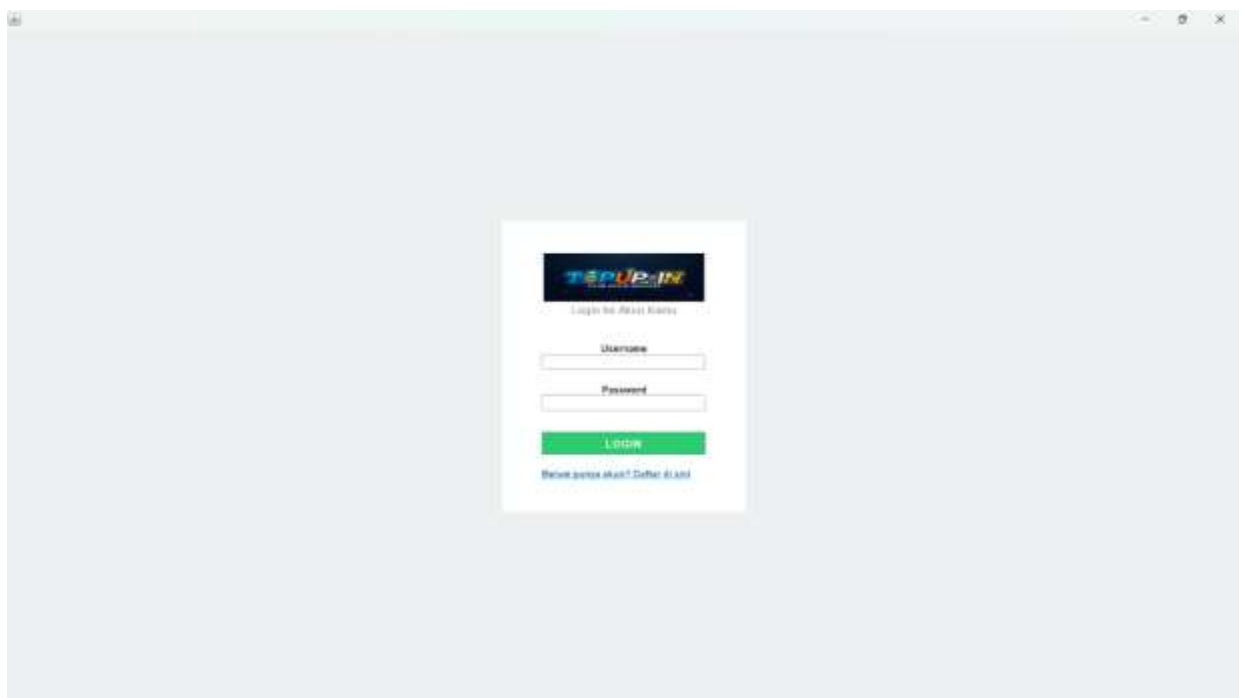
Gambar 2. 8 UI Login
