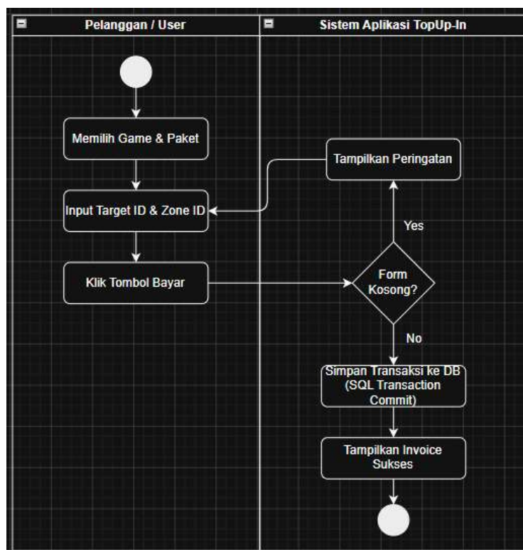
Gambar 2. 4 Transaksi
