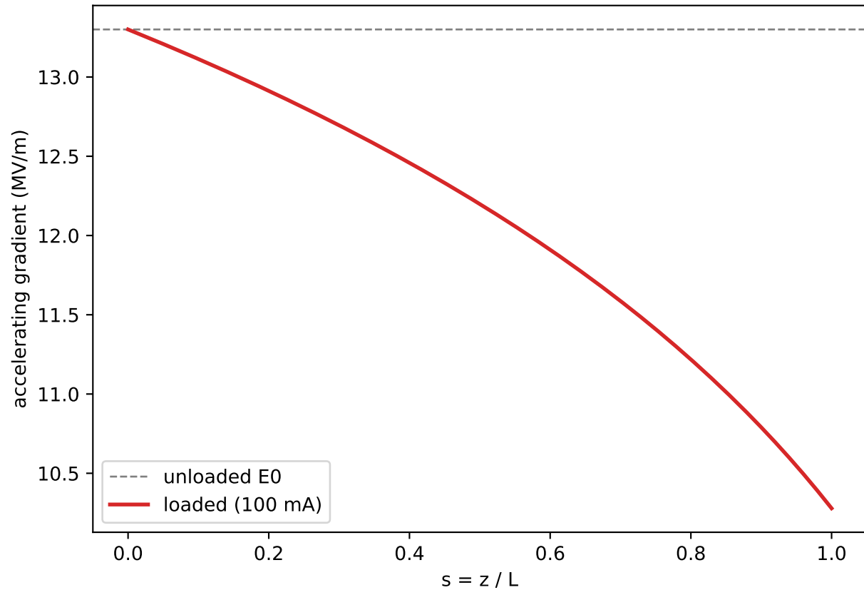
Loaded gradient sag (CG, 100 mA)
