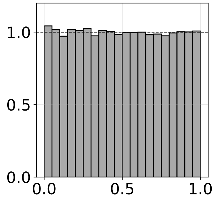
n = 5000
