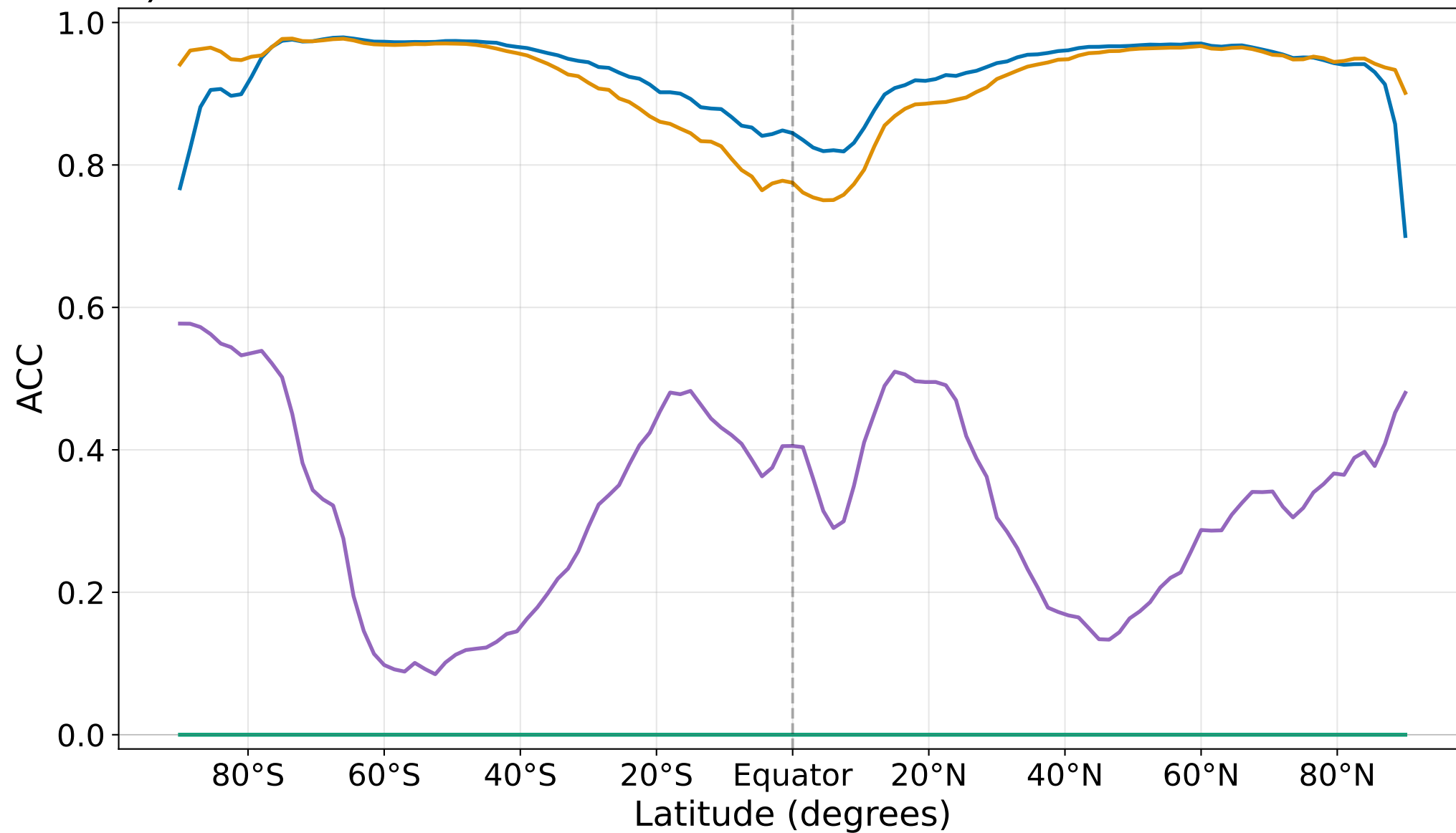
e) ACC
