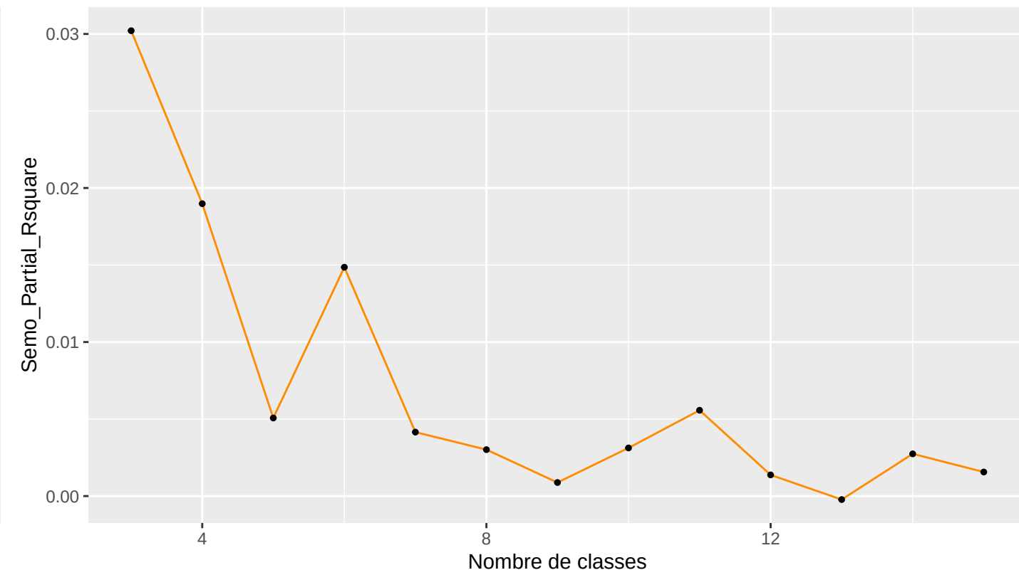
Coefficient Semi_Partial_Rsquare en fonction du nombre de centres de clusters.
