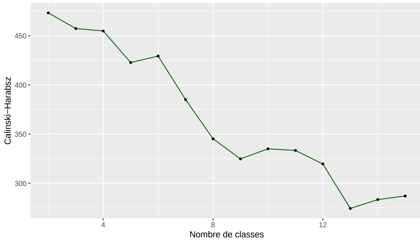
Coefficient de Calinski-Harabsz en fonction du nombre de centres de clusters.
