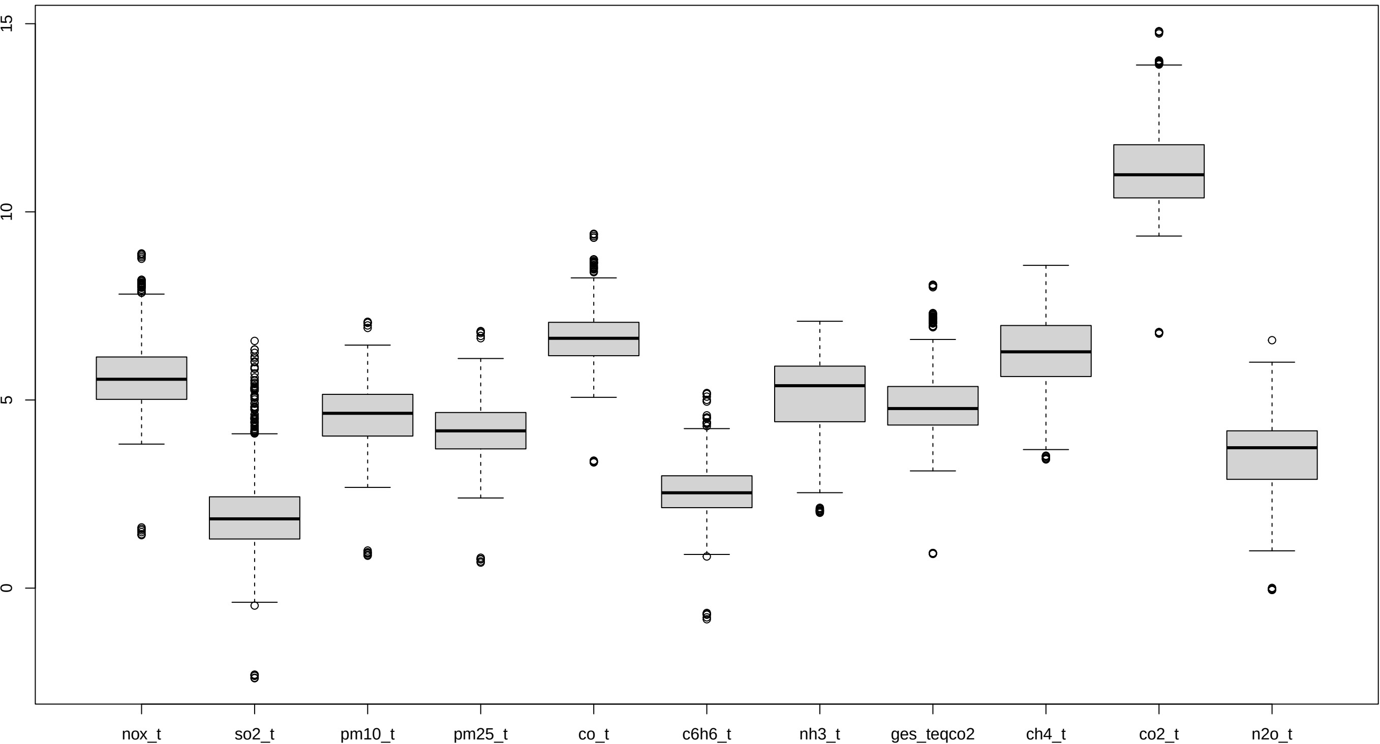
Boxplot de nos variables quantitaves
